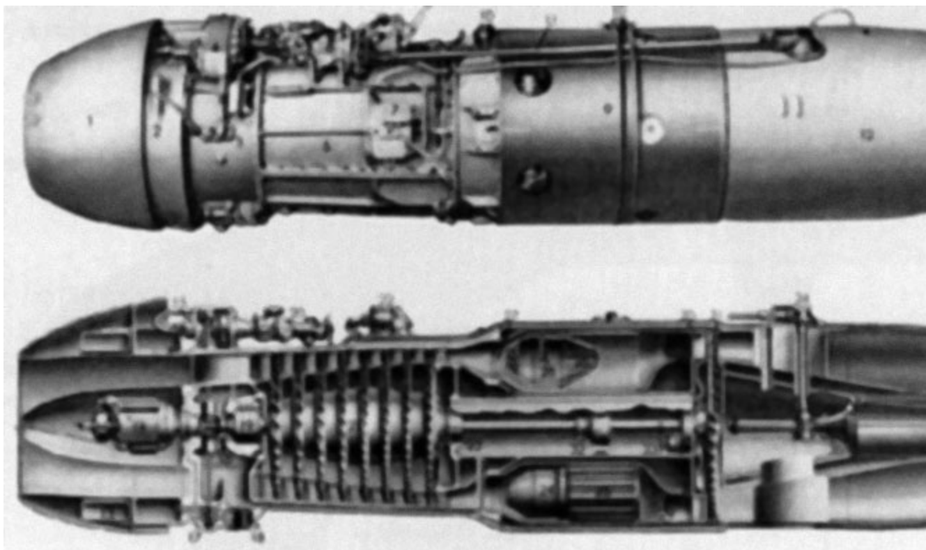
Компоновка первого ТРД концерна «Юнкерс» Jumo 004
