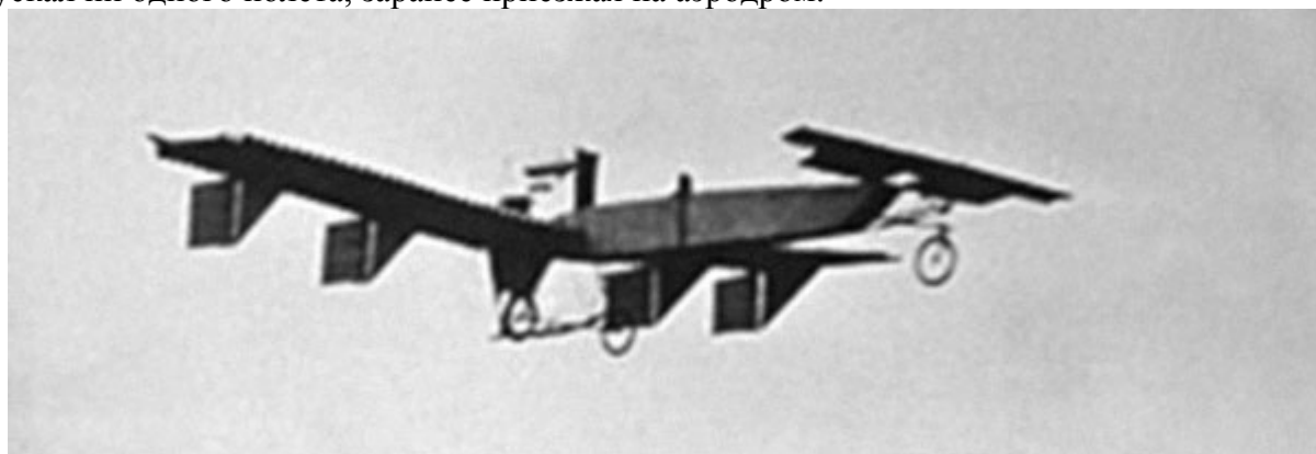
Модифицированная «утка» Райснера, 1913 г.
