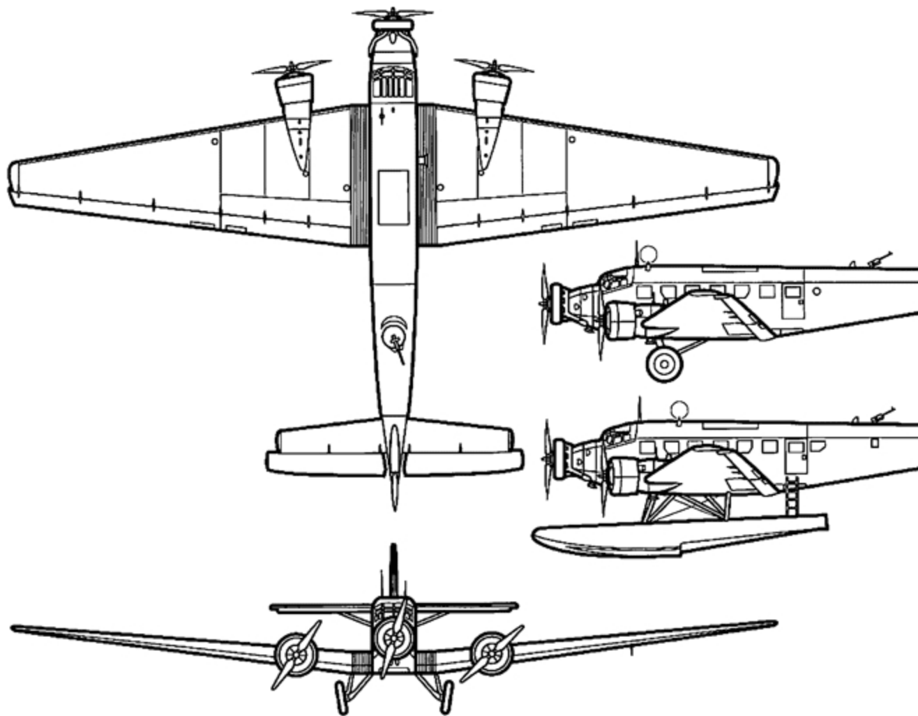
Общий вид улучшенного самолета Юнкерса Ju-52, 1932 г.
