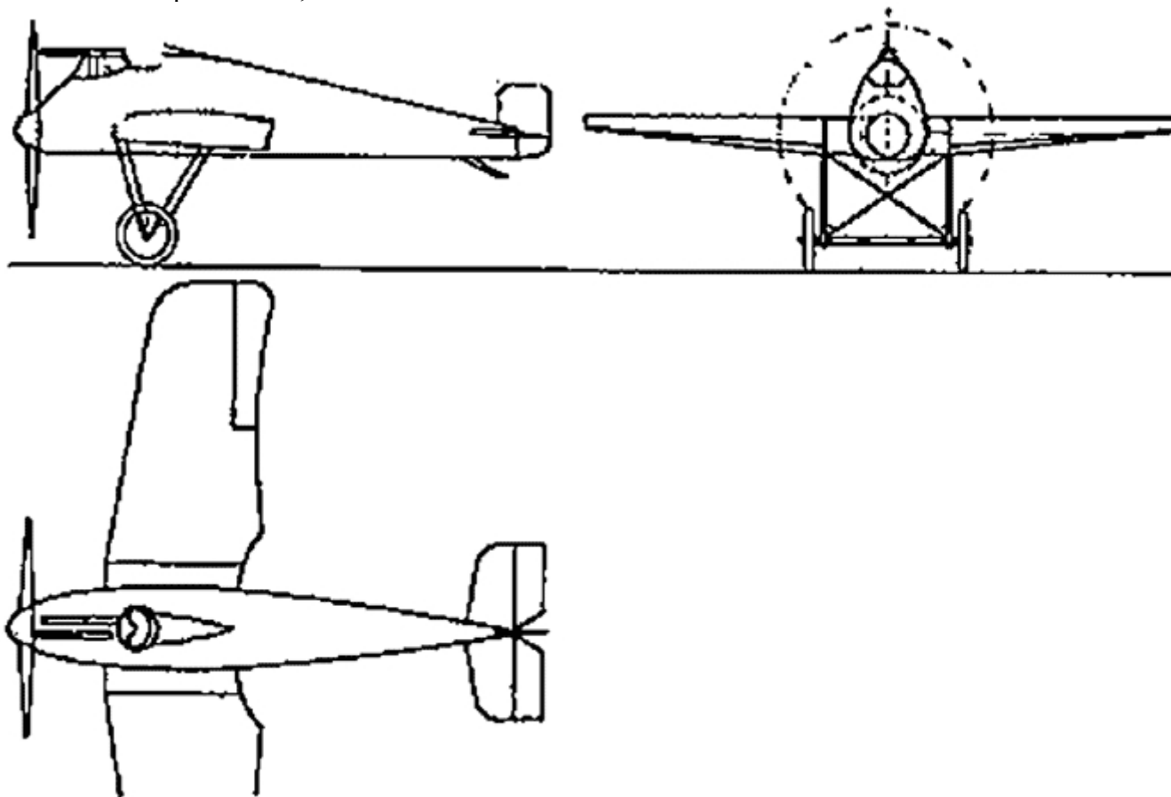
Проект истребителя Юнкерса J-5, 1917 г.
