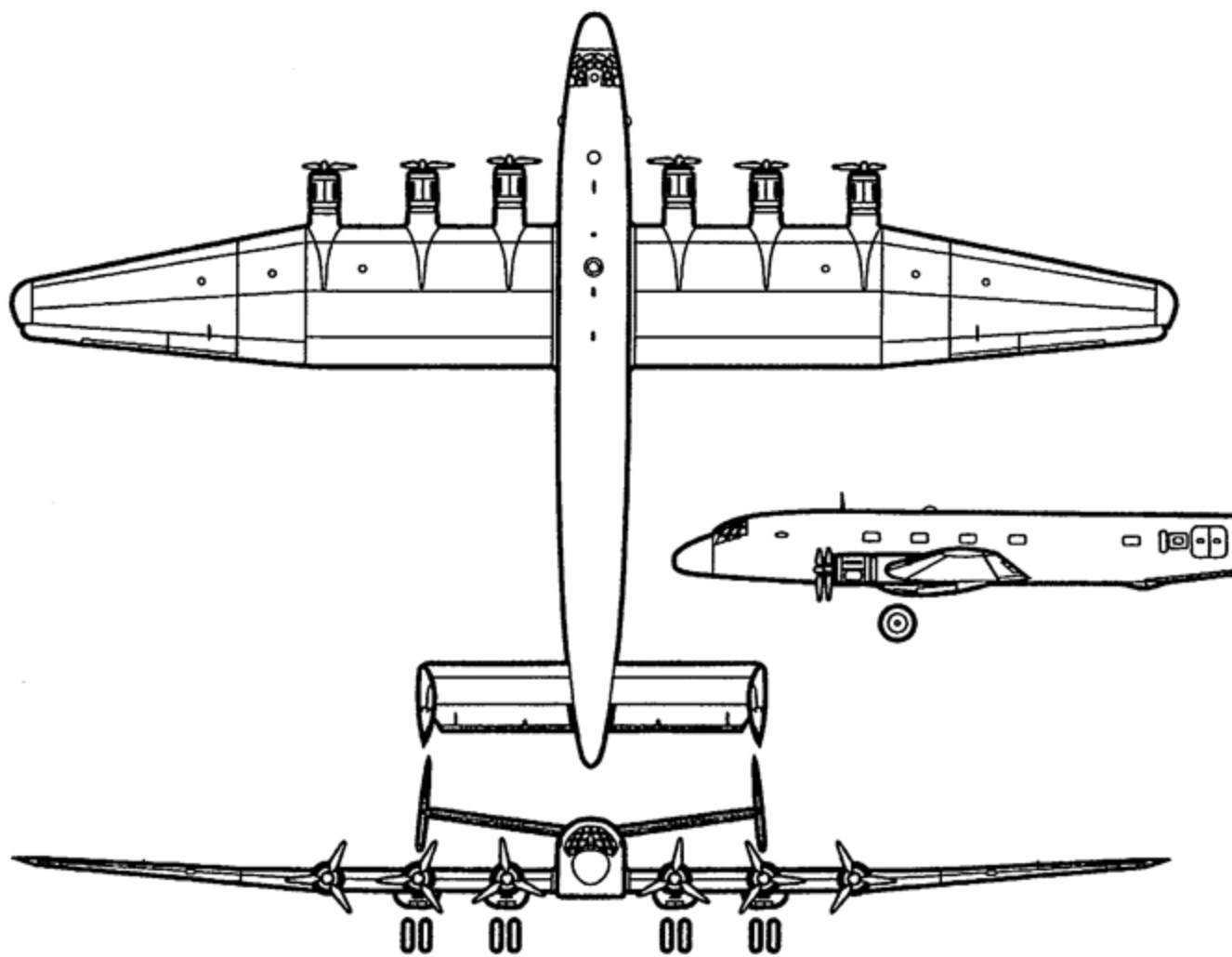
Общий вид дальнего бомбардировщика Ju-390, 1942 г.
