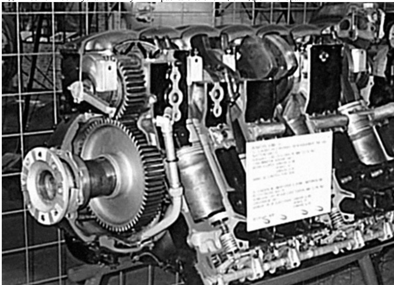
Јумо 211 в разрезе
