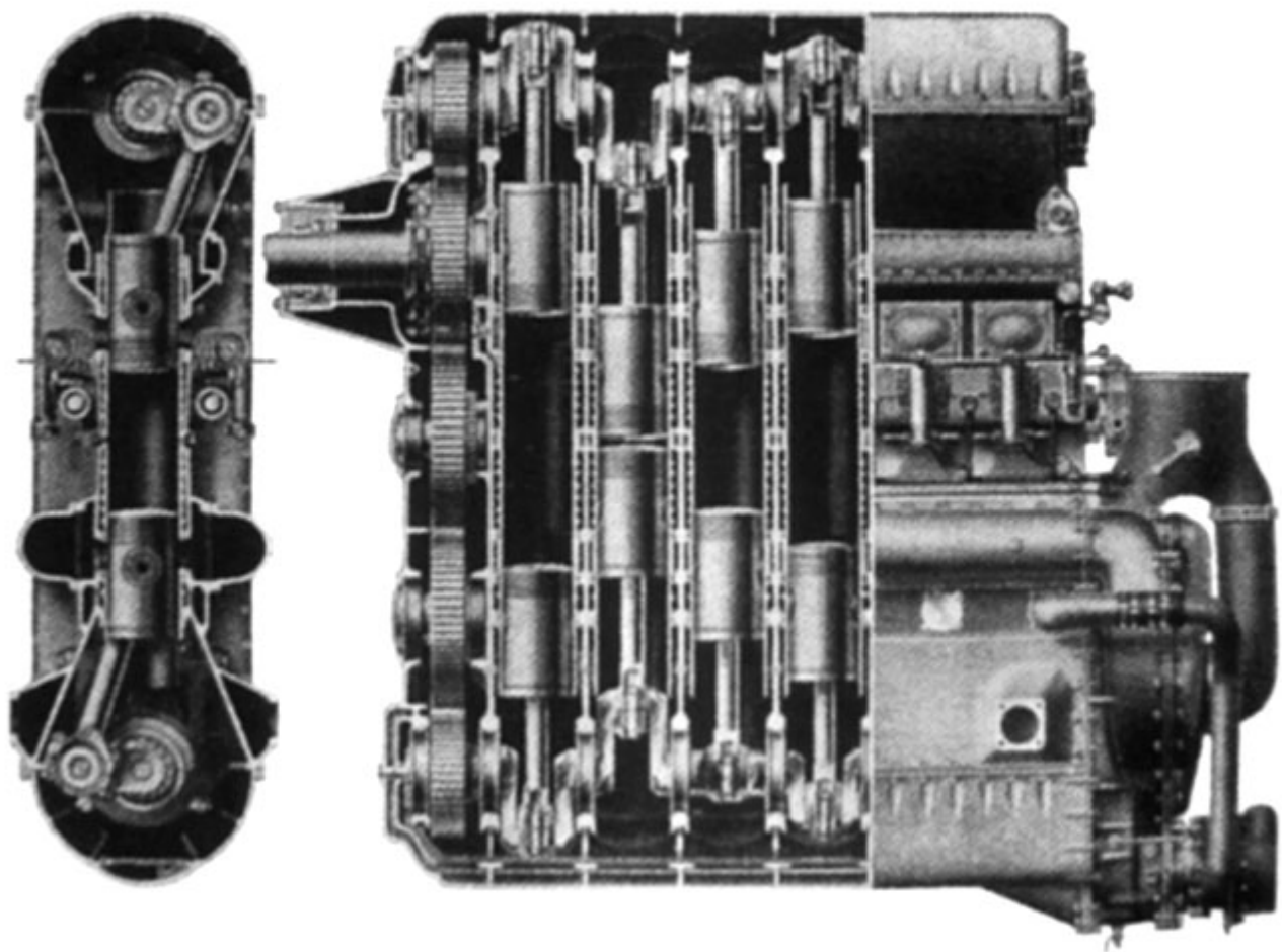
Дизель Юнкерса Jumo 4, 1930 г.
