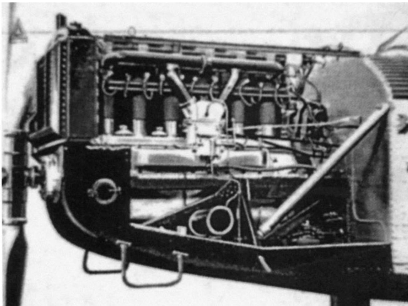
Двигатель Юнкера L5 – «сердце» его пассажирского F-13
