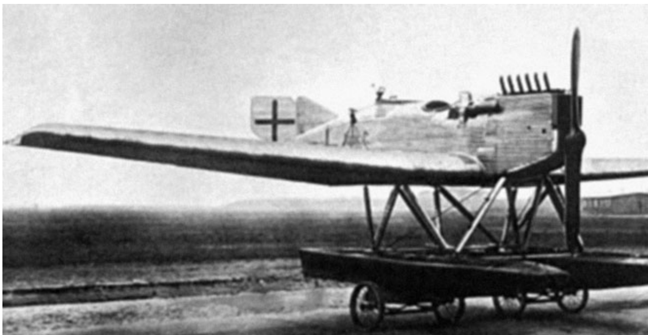
Морской двухместный разведчик и спасатель J-11, 1918 г.
