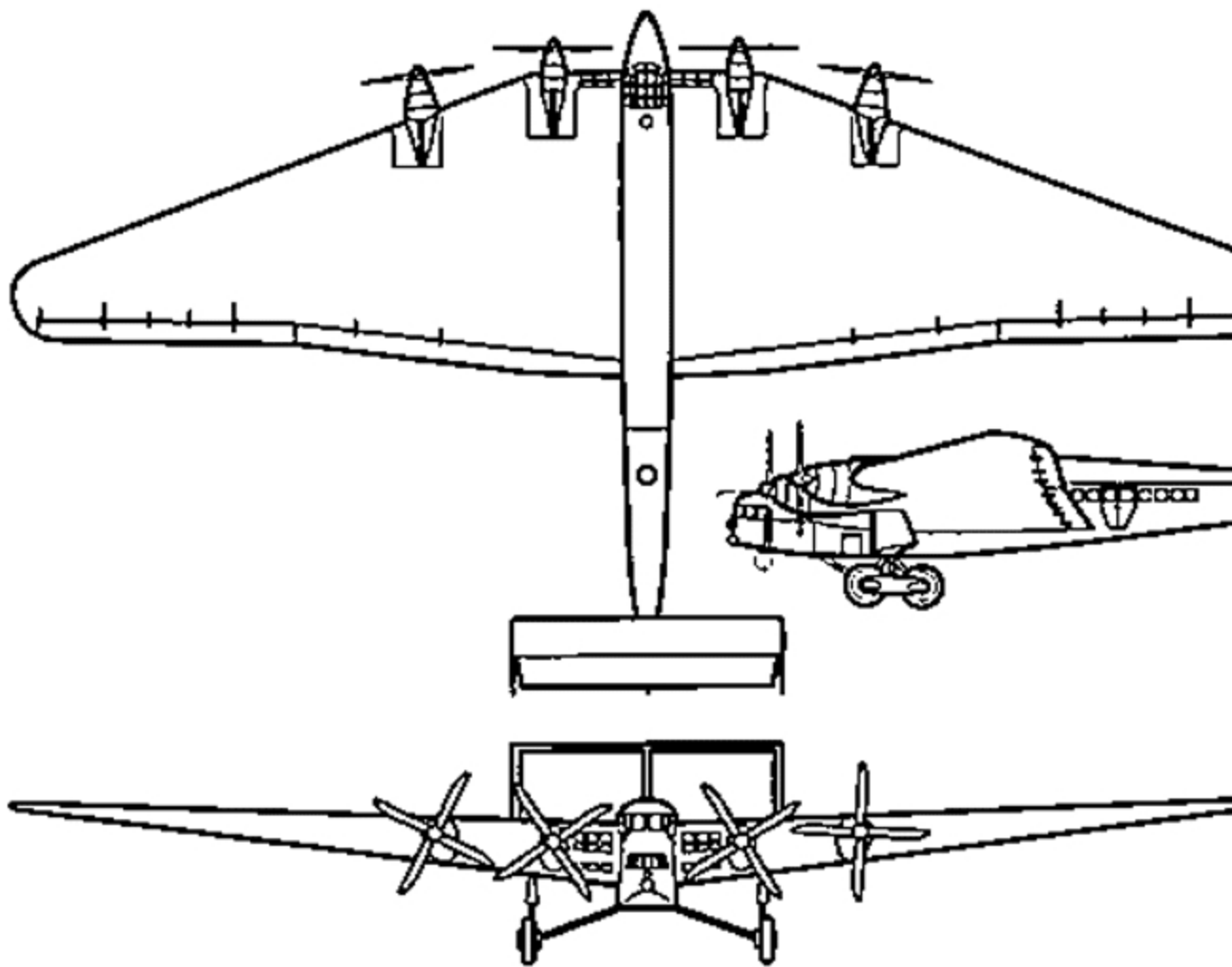
Общий вид второго гиганта Юнкерса G-38се
