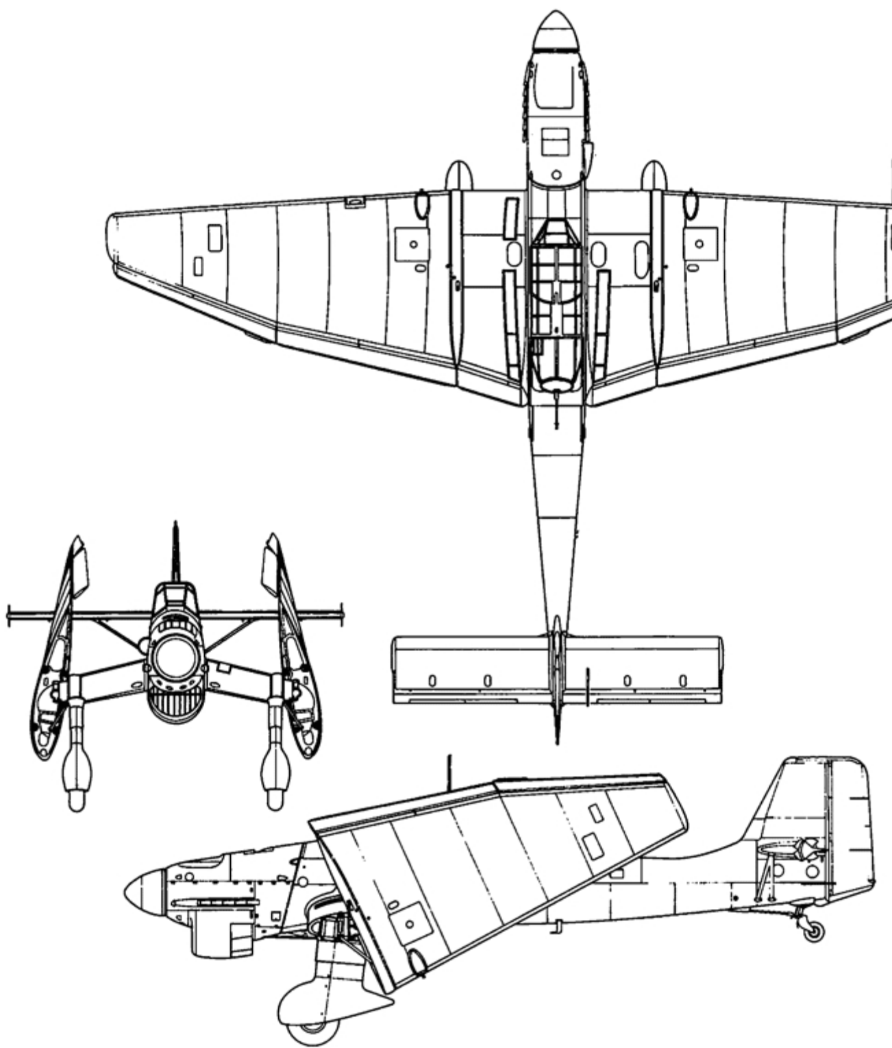
Общий вид палубного Ju-87 С, 1939 г.
