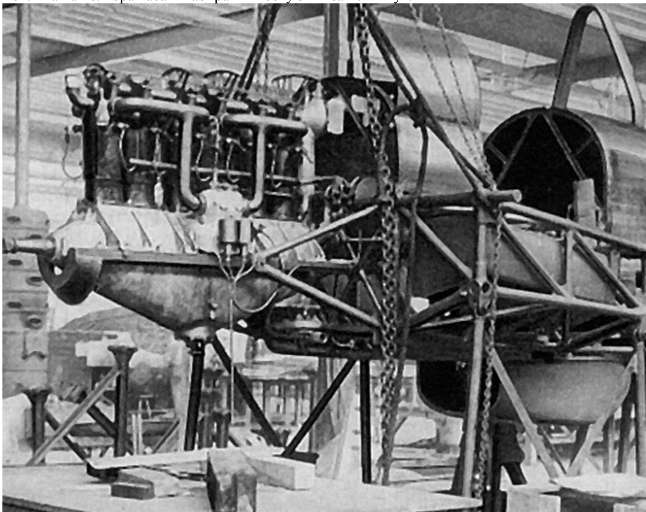
Центральная ферма истребителя Юнкерса J-2
