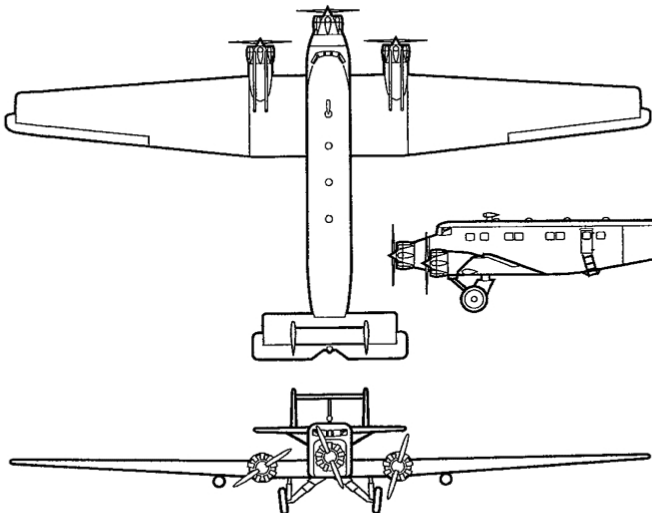
Пассажирский G-31 с радиальными моторами, 1928 г.
