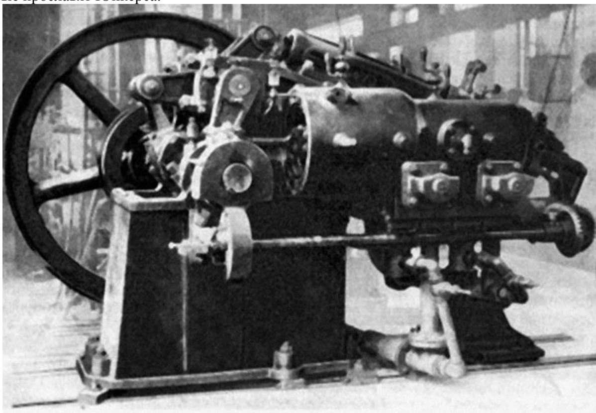
Опытный мотор Юнкерса M11, 1904 г.
