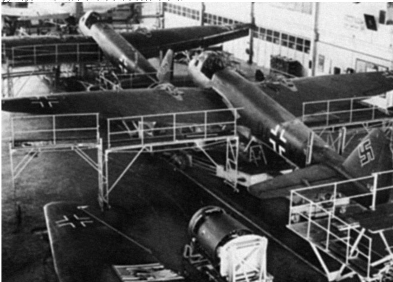
Конвейер на заводе общей сборки в Бернбурге
