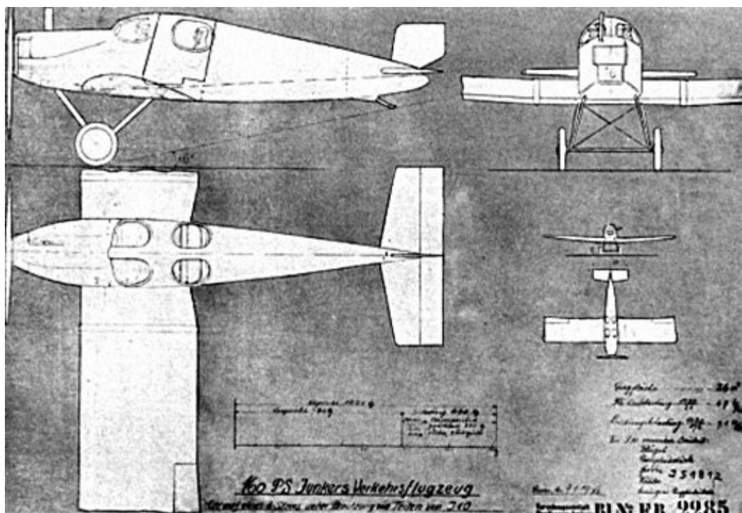
Забракованный проект пассажирского самолета J-12
