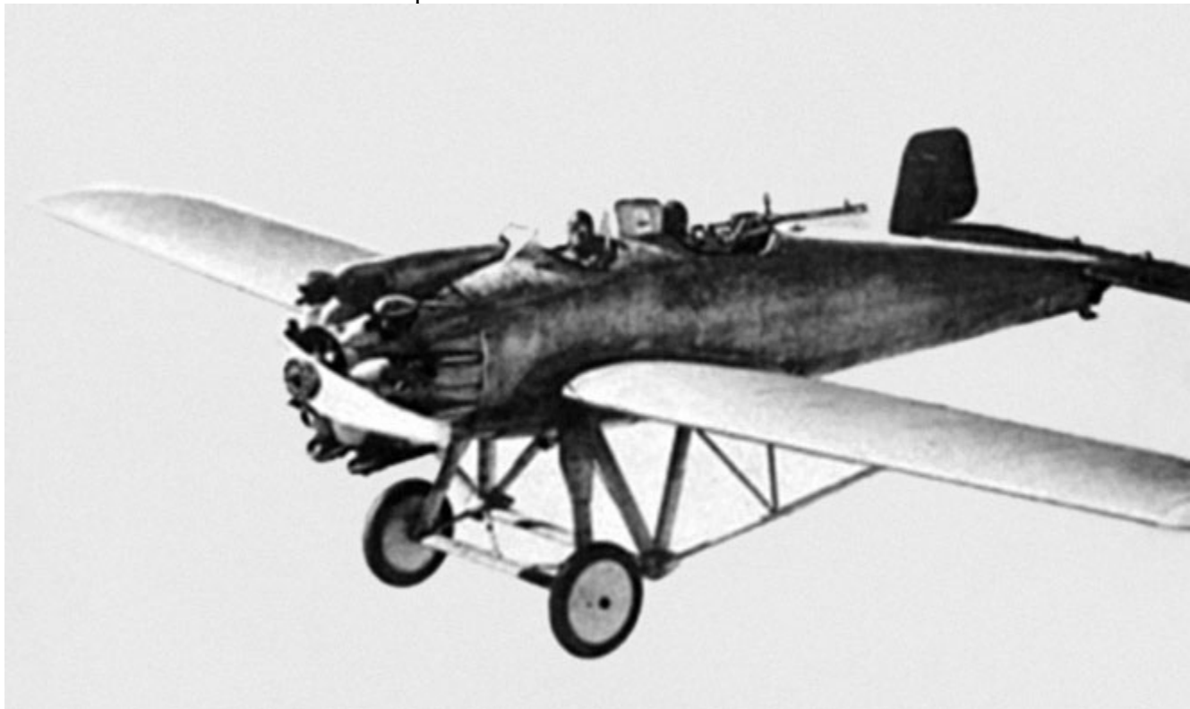
Истребитель Юнкерса К-47, 1929 г.
