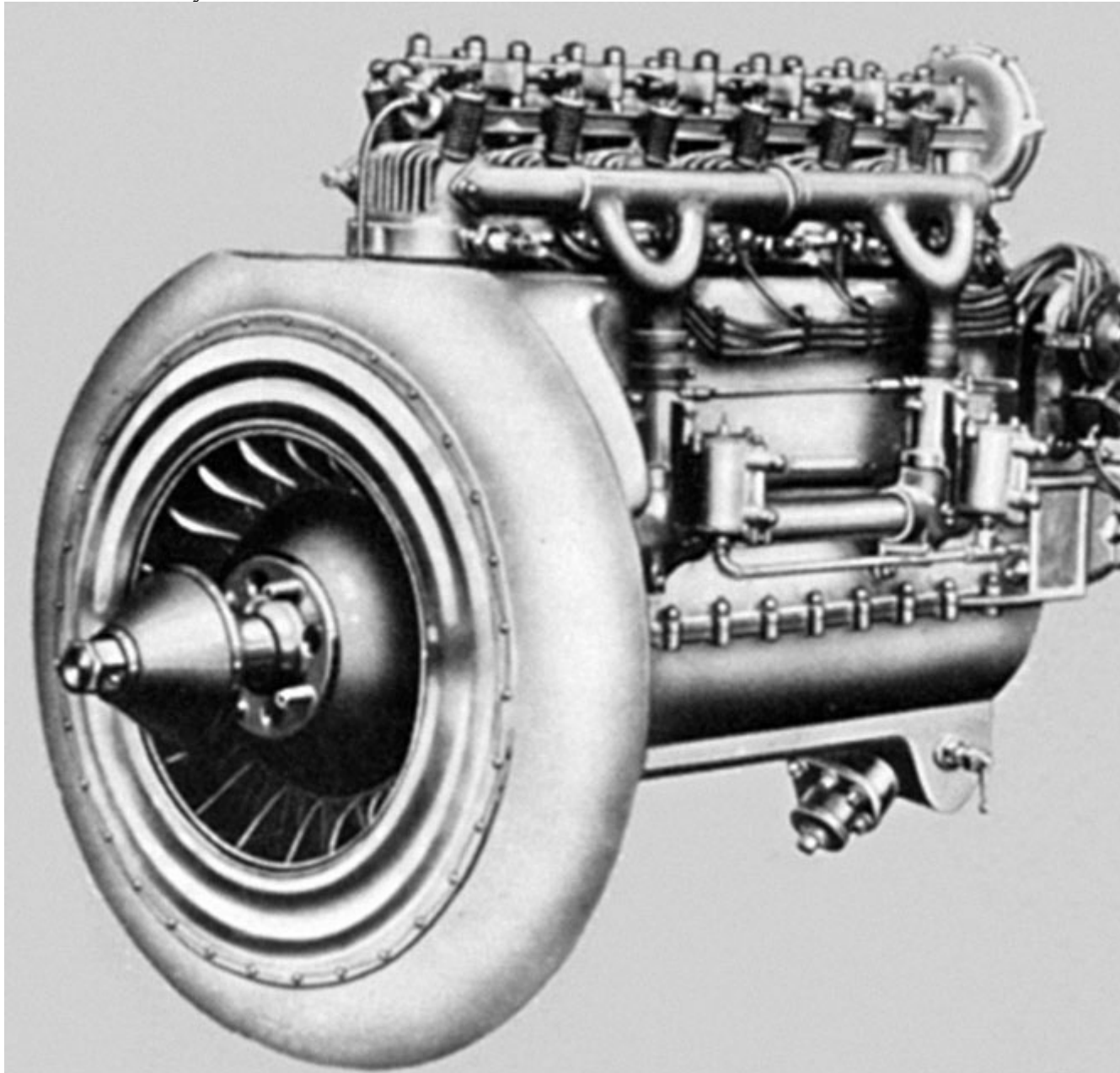
Авиационный мотор Юнкерса L1
