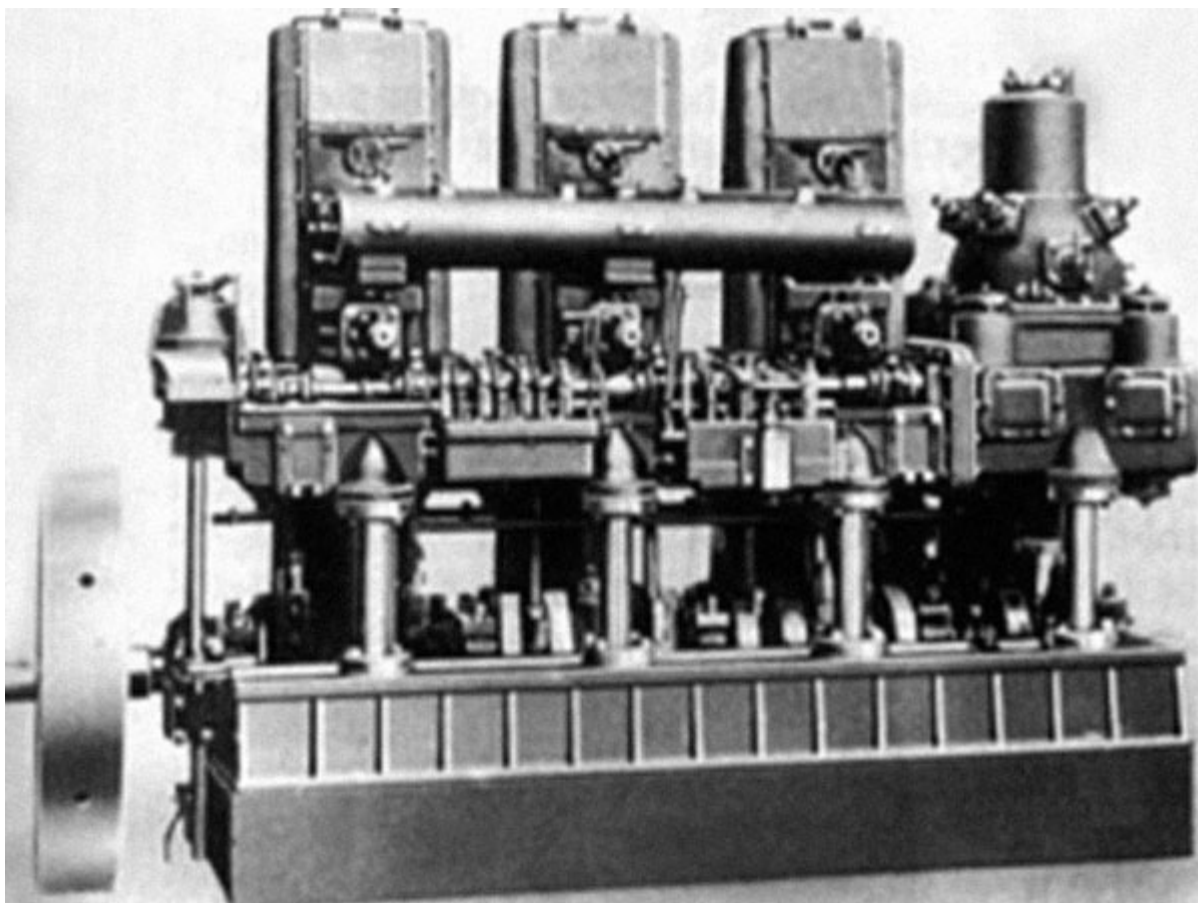
Лицензионный судовый двигатель Юнкерса, 1911 г.
