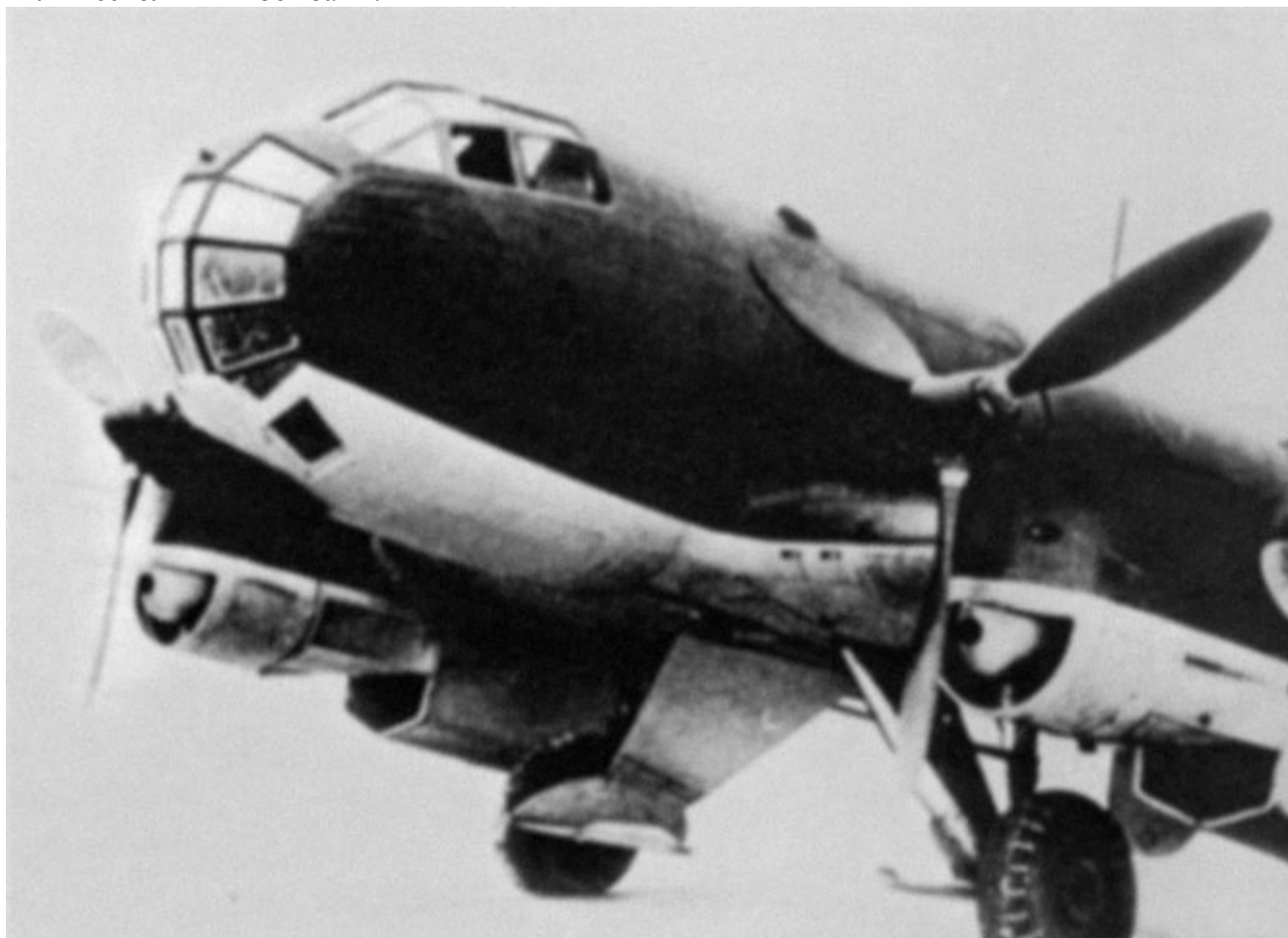
Гермокабина высотного разведчика «юнкерс» 86Р, 1940 г.
