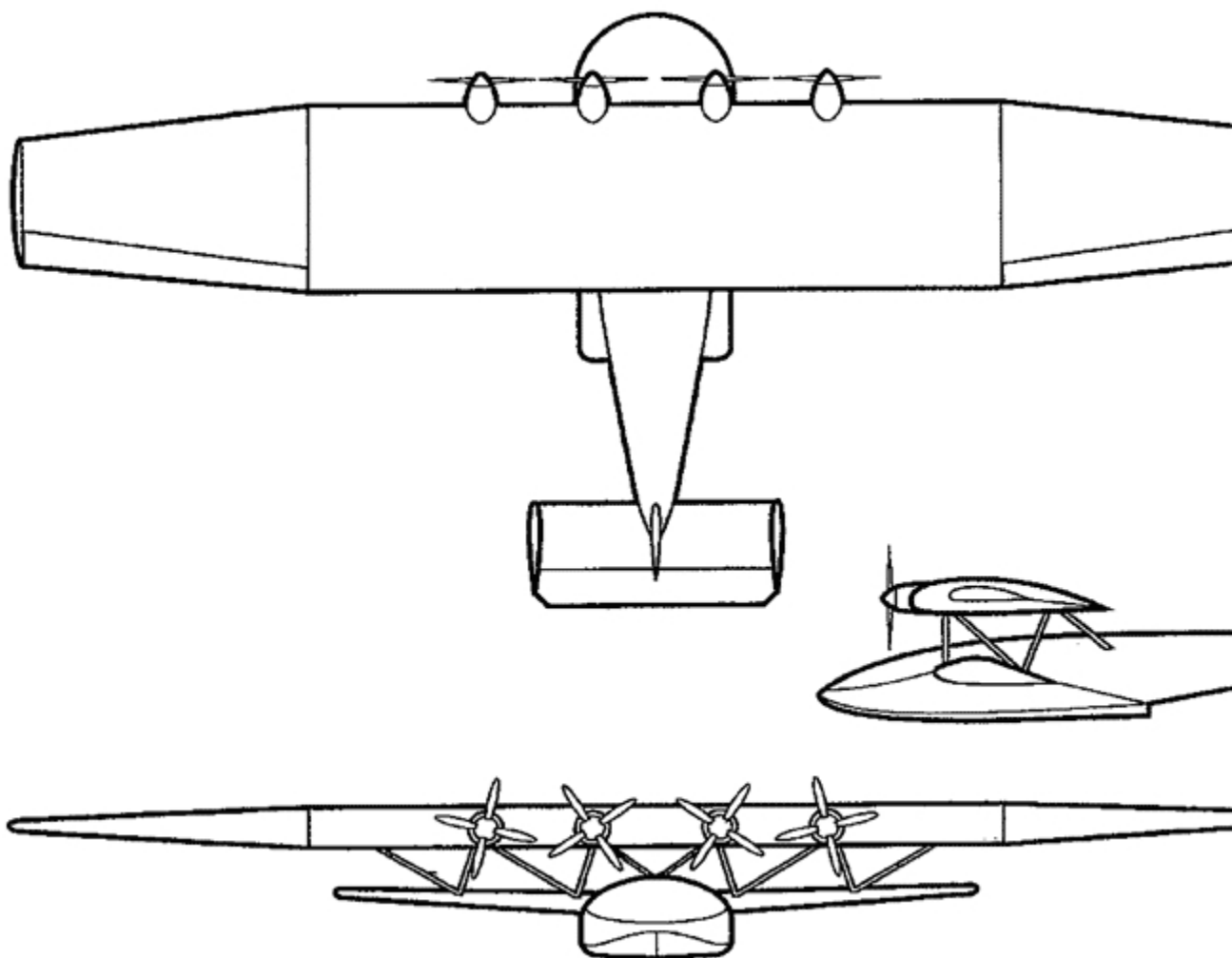
Проект летающей лодки Flugboot F, 1918 г.
