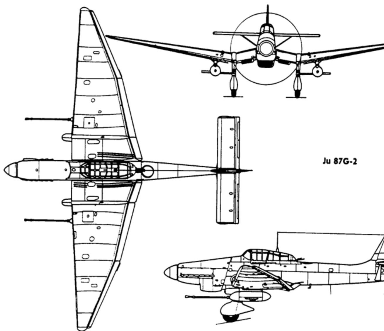
Общий вид серийной модификации Ju-87 G-2
