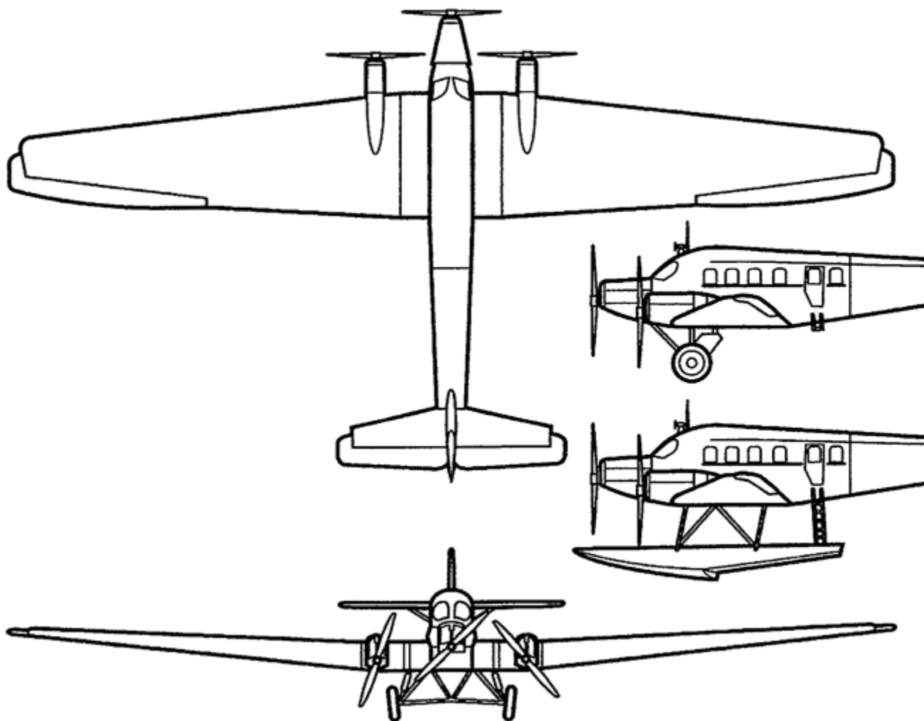
Общий вид пассажирского самолета Юнкерса G-23, 1924 г.
