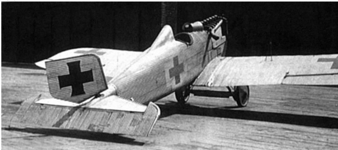
Опытный истребитель Юнкерса J-7, 1917 г.
