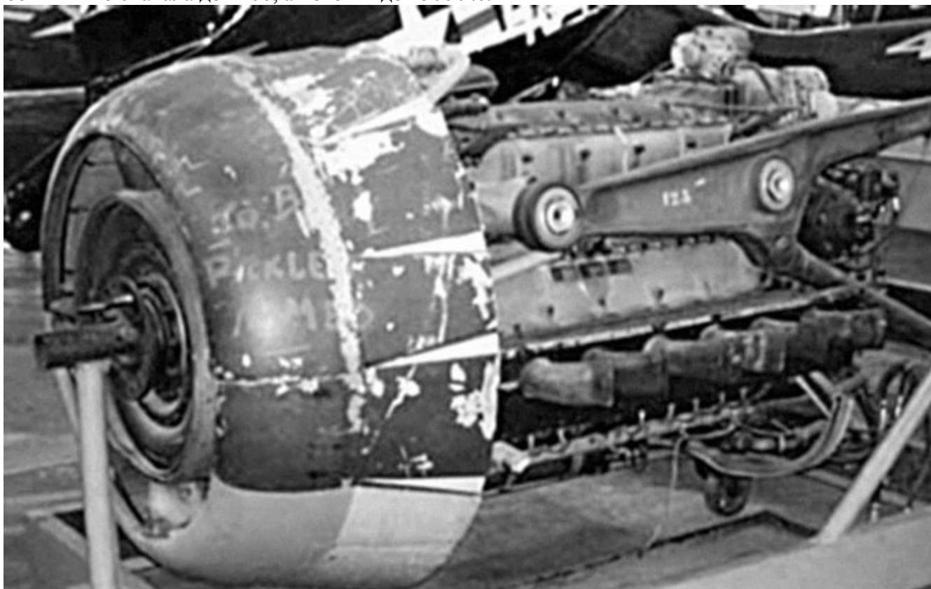
Кольцевые радиаторы мотора концерна «Юнкерс»
