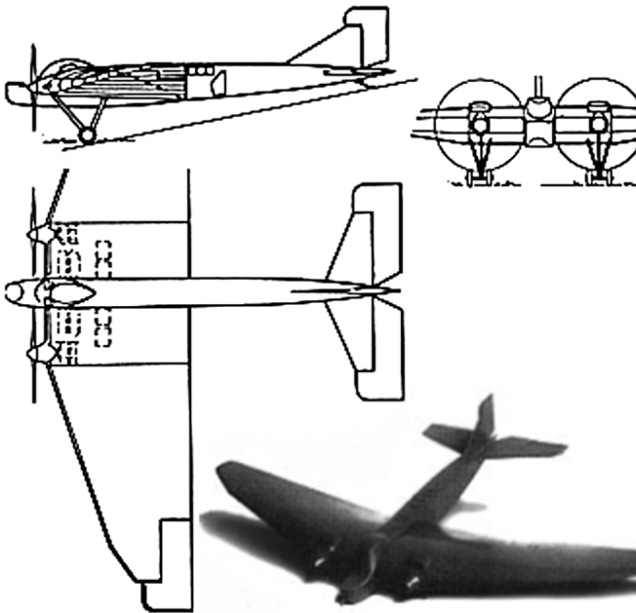
Проект R I бомбардировщика Юнкерса, 1917 г.
