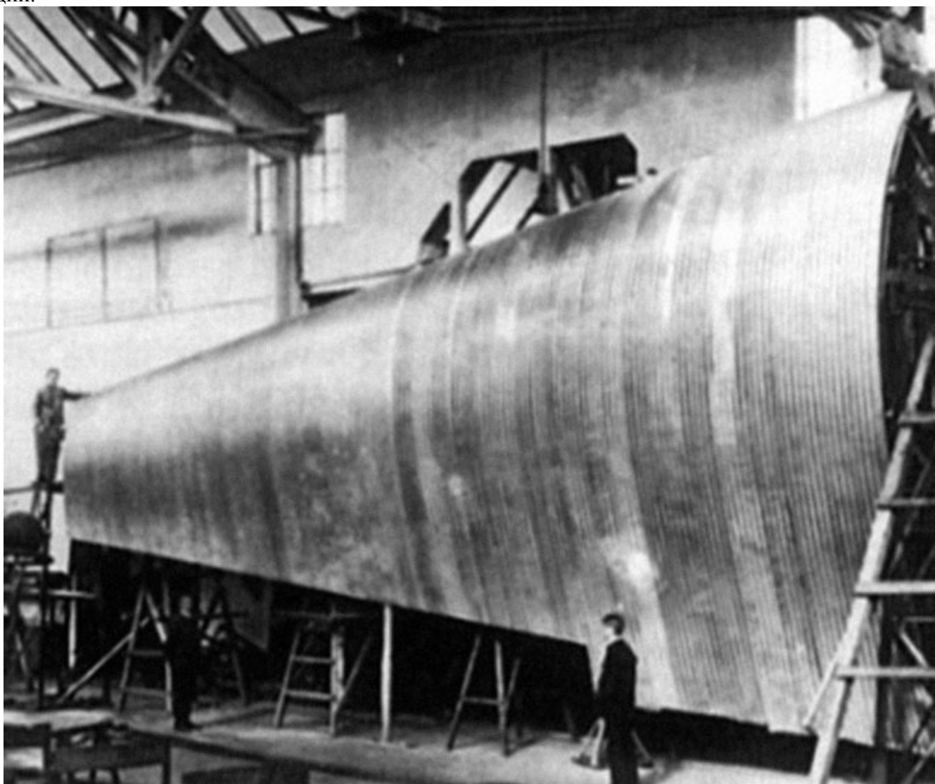
Крыло лайнера Юнкерса JG-1, 1921 г.
