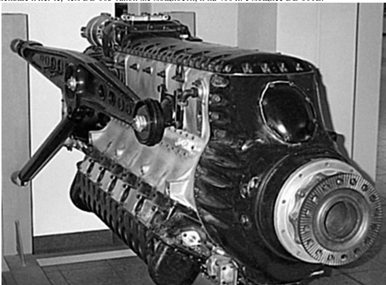
12-цилиндровый Jumo 213 мощностью 1750 л.с.
