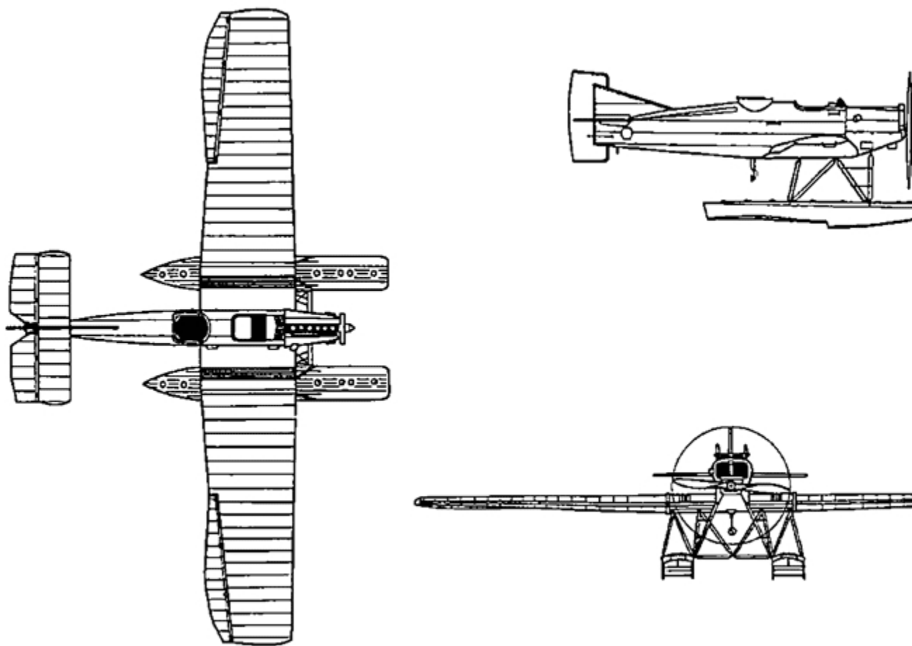
Общий вид морского разведчика Юнкерса J-20, 1922 г.
