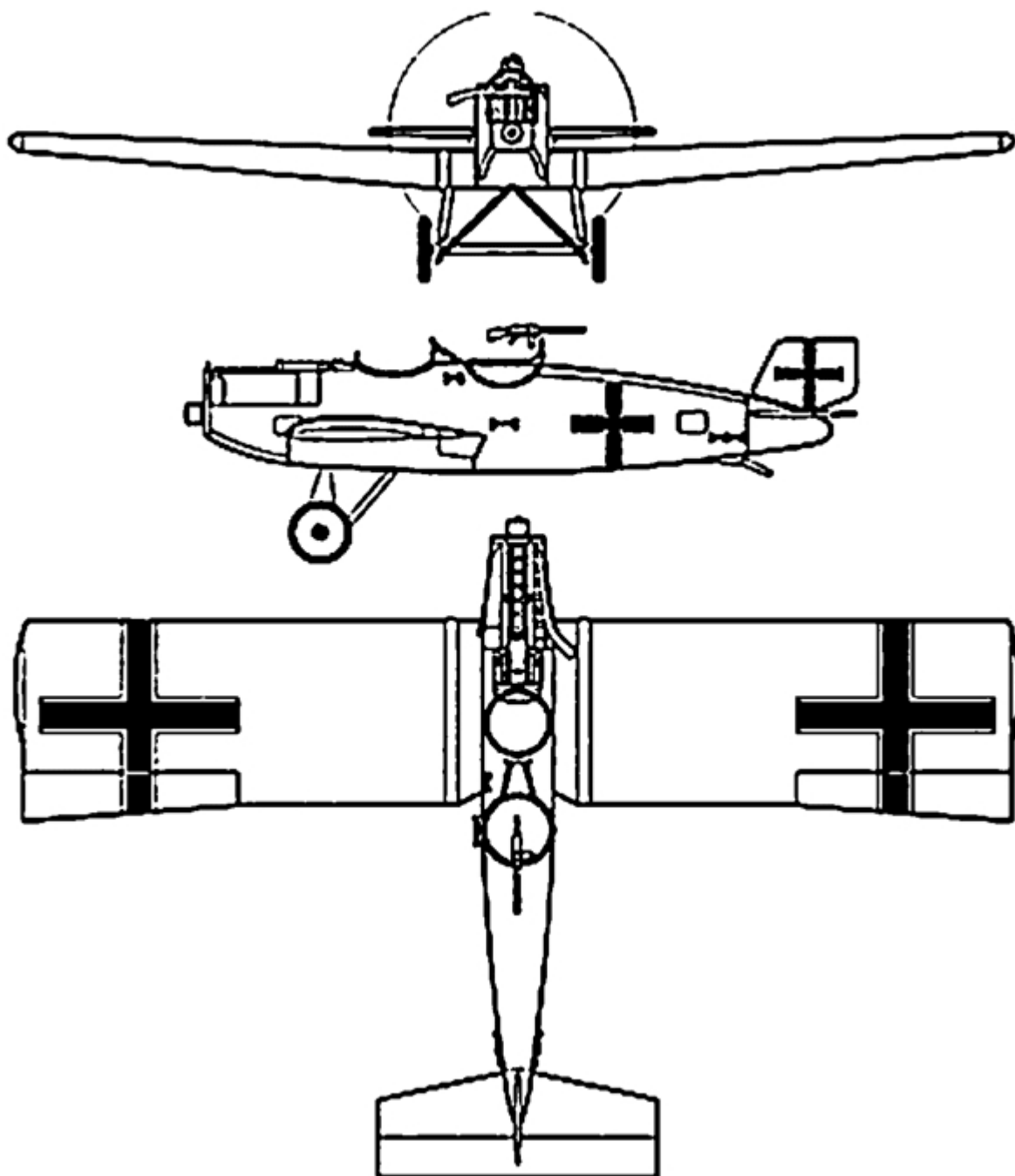
Двухместный многоцелевой Junk CL.I, 1918 г.
