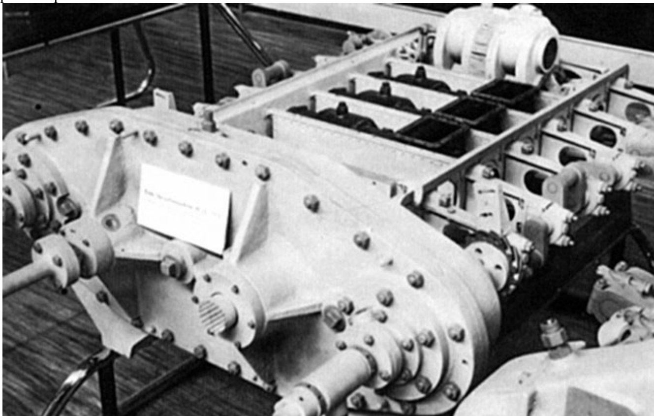
Первый авиационный экспериментальный мотор Юнкерса Мо3
