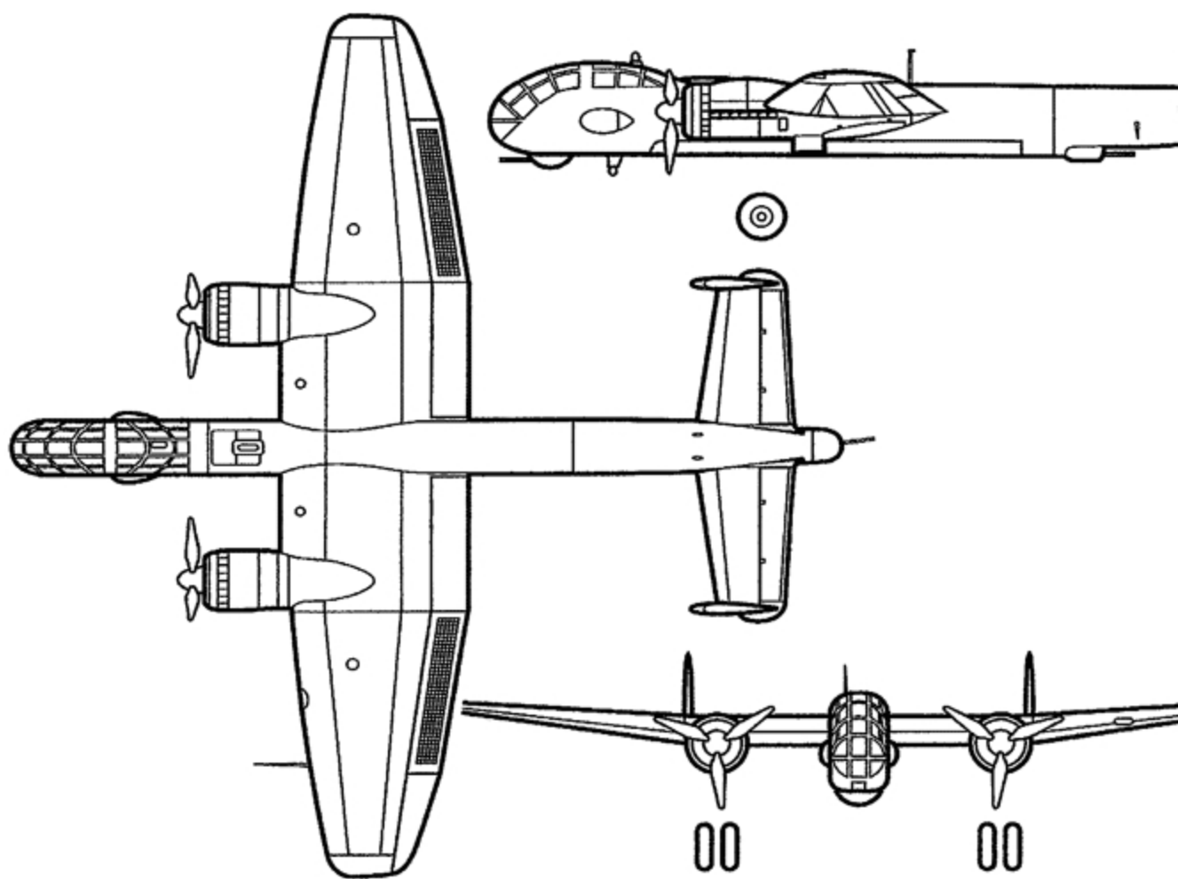
Проект бомбардировщика профессора Хертеля, 1940 г.
