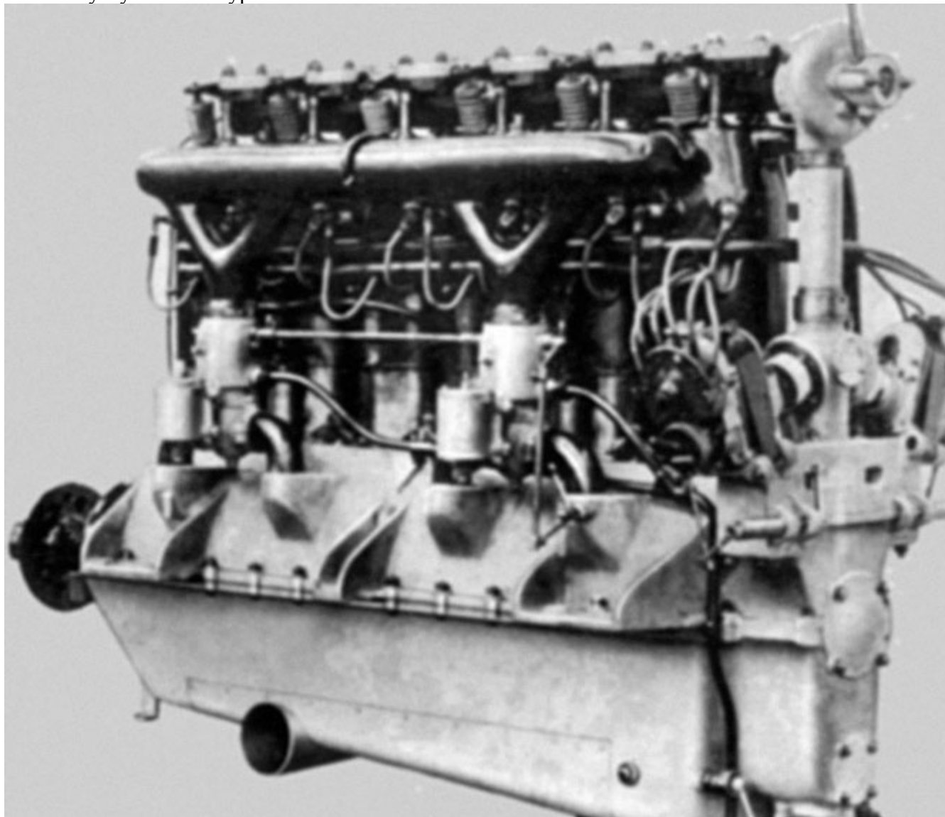
Серийный авиадвигатель Юнкерса L2, 1924 г.
