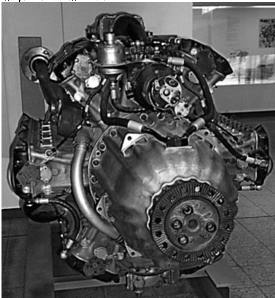
Несостоявшийся мотор Jumo 222
