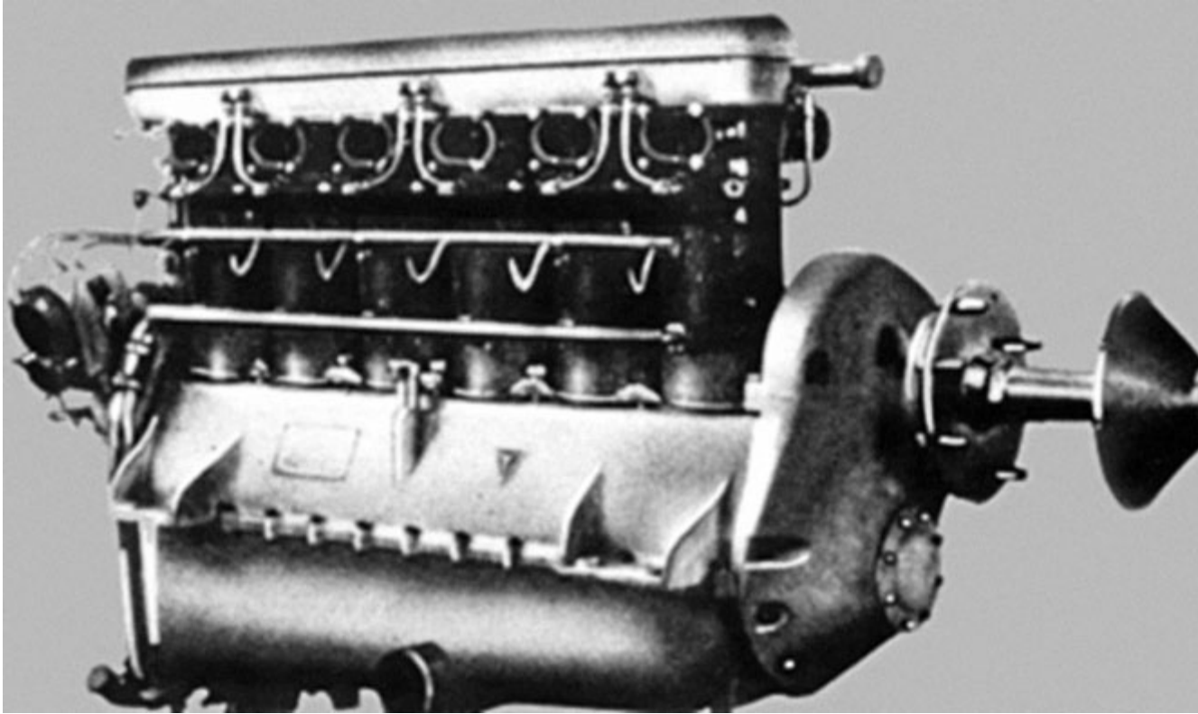
Редукторный авиационный мотор Юнкерса L8, 1928 г.
