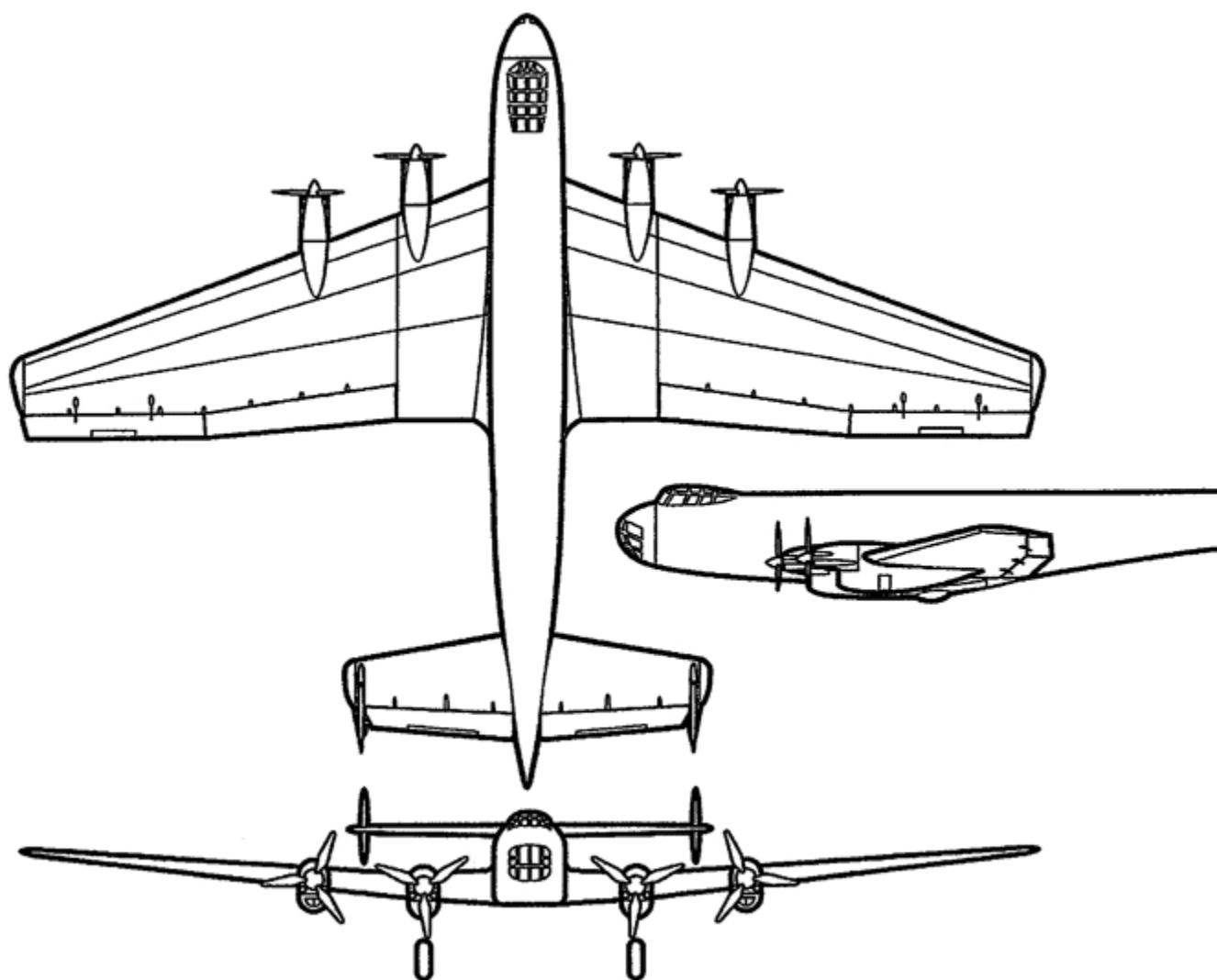
Общий вид дальнего бомбардировщика Ju-89, 1936 г.
