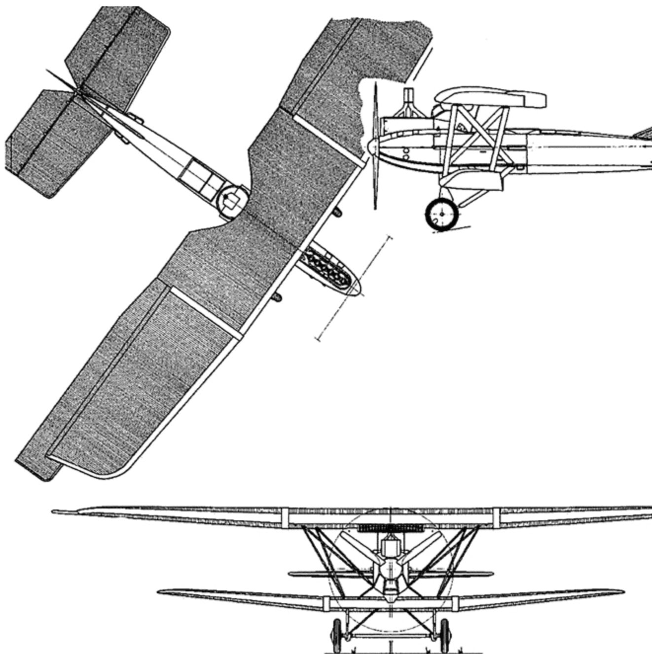
Общий вид серийного дюралевого самолета Юнкера, 1917 г.
