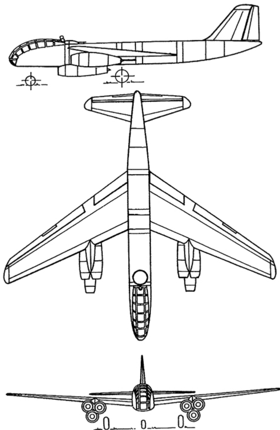
Проект бомбардировщика EF-131, 1946 г.
