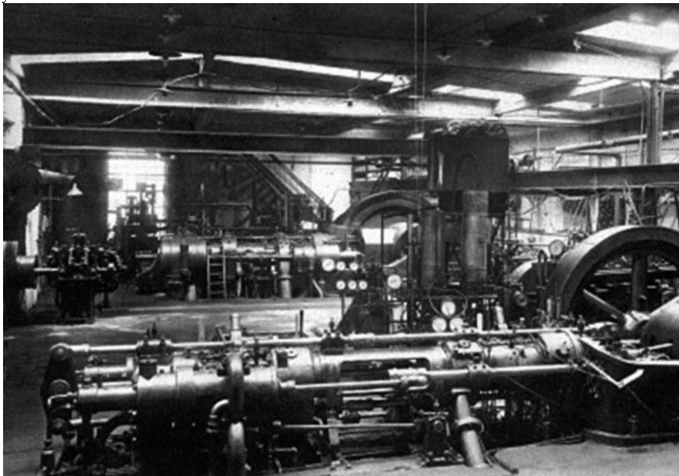
Двигатель Юнкерса M12 в машинном зале в Ахене
