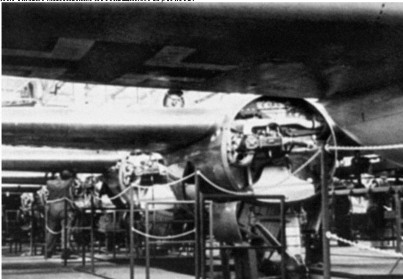
Конвейер сборки на заводе крыльев в Хальберштадте
