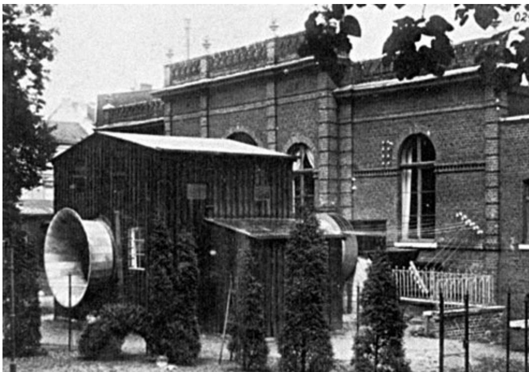
Аэродинамическая труба Юнкера во дворе его дома, 1914 г.
