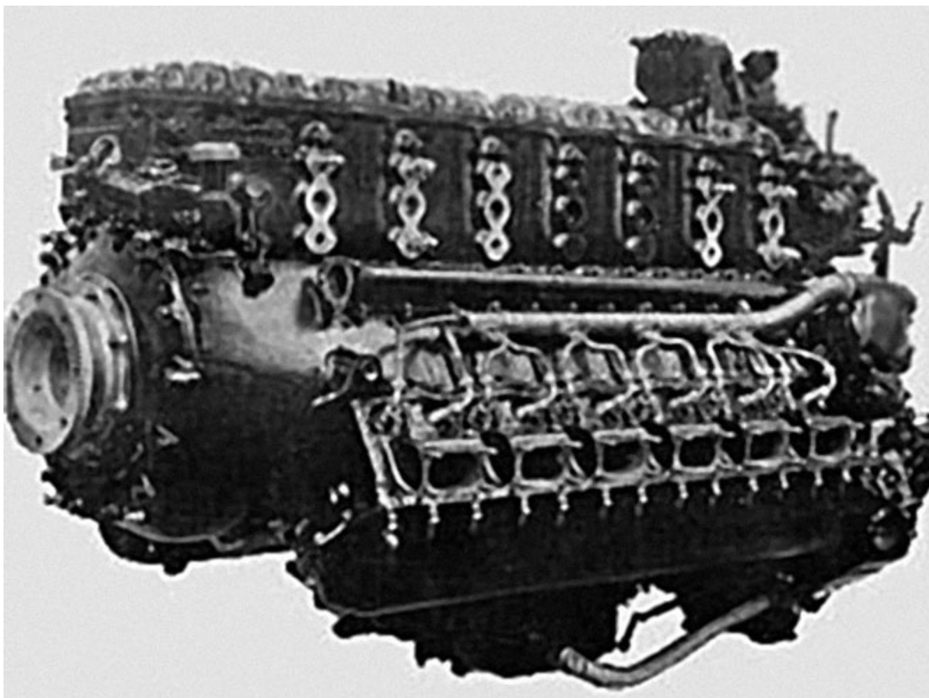
Перевернутый мотор Юнкерса Jumo 210
