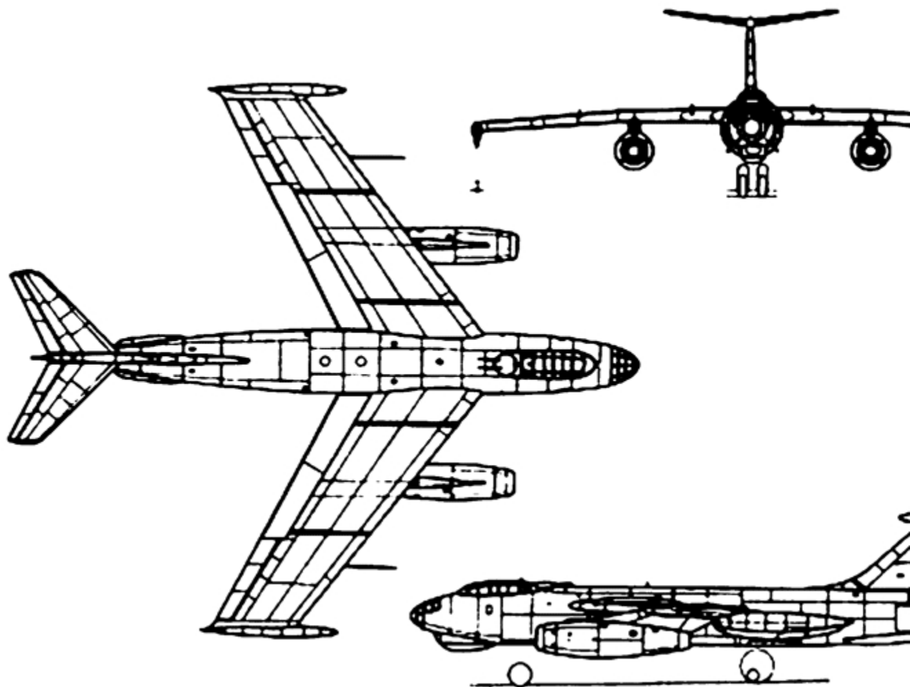
Общий вид бомбардировщика «150», 1949 г.
