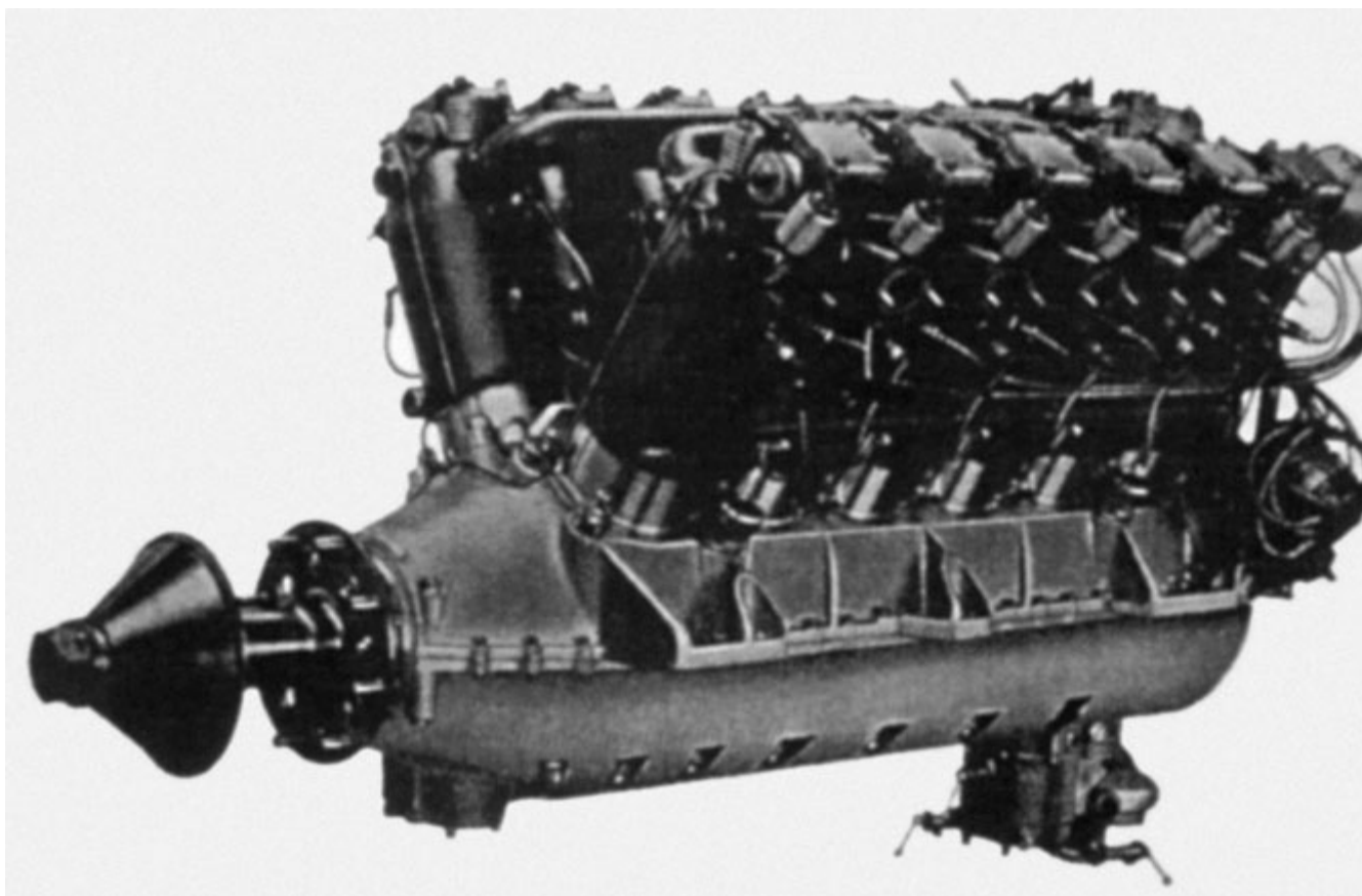
Мотор Юнкерса L55, 1927 г.
