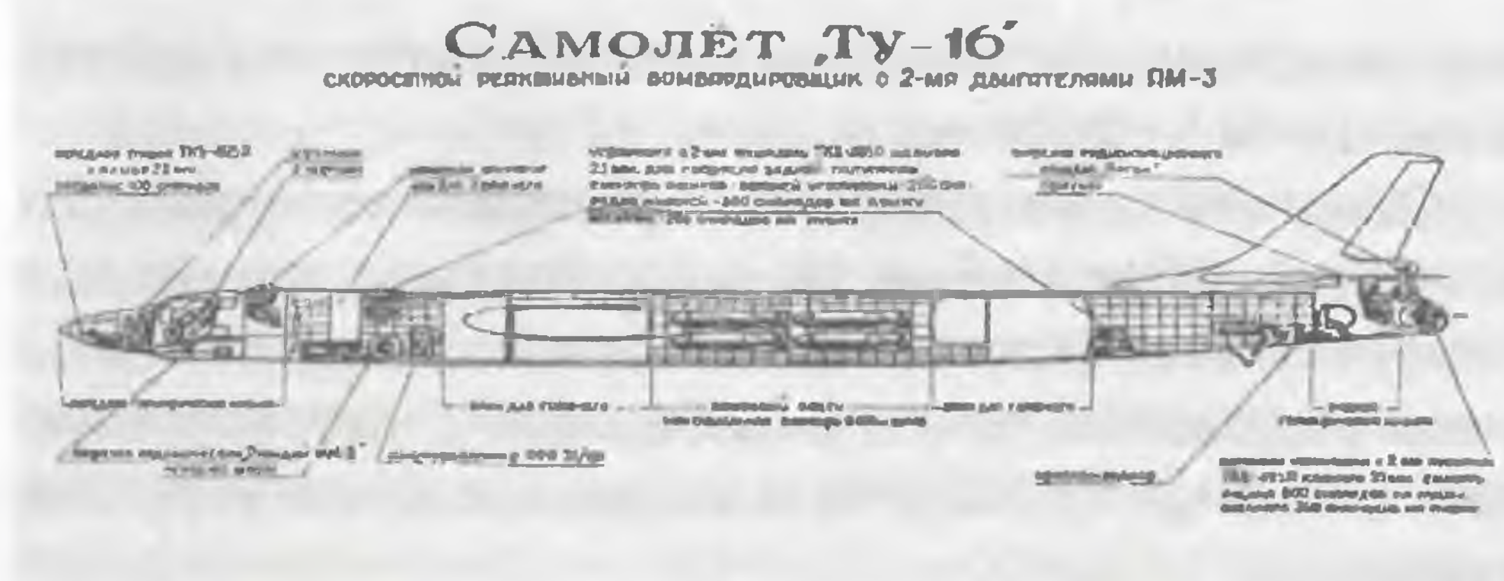
Компоновка Ту-16 (Ту-88)
