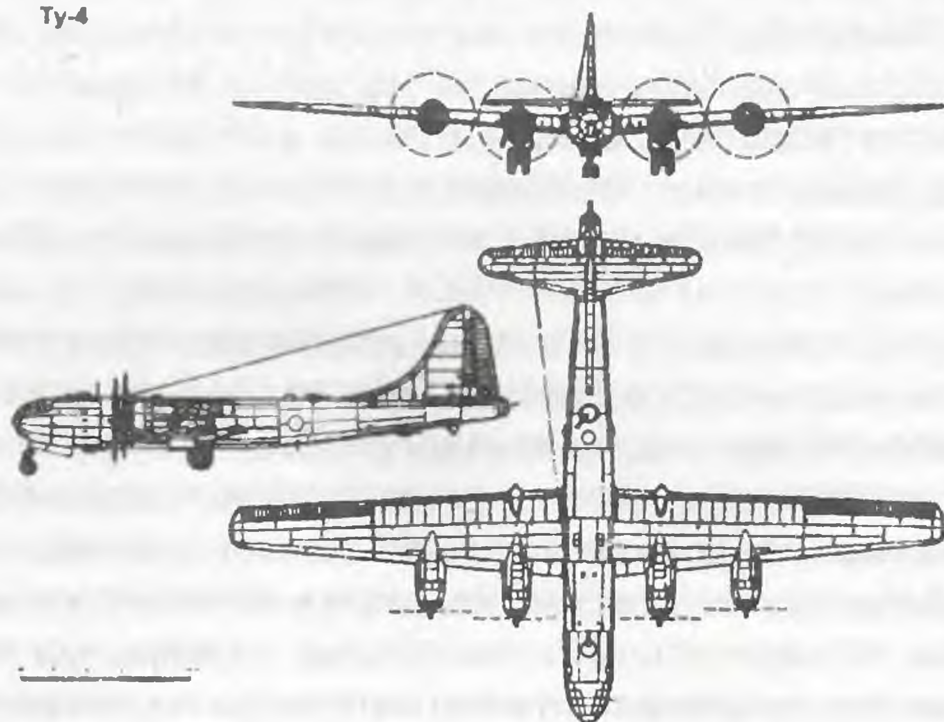
Ту-4
