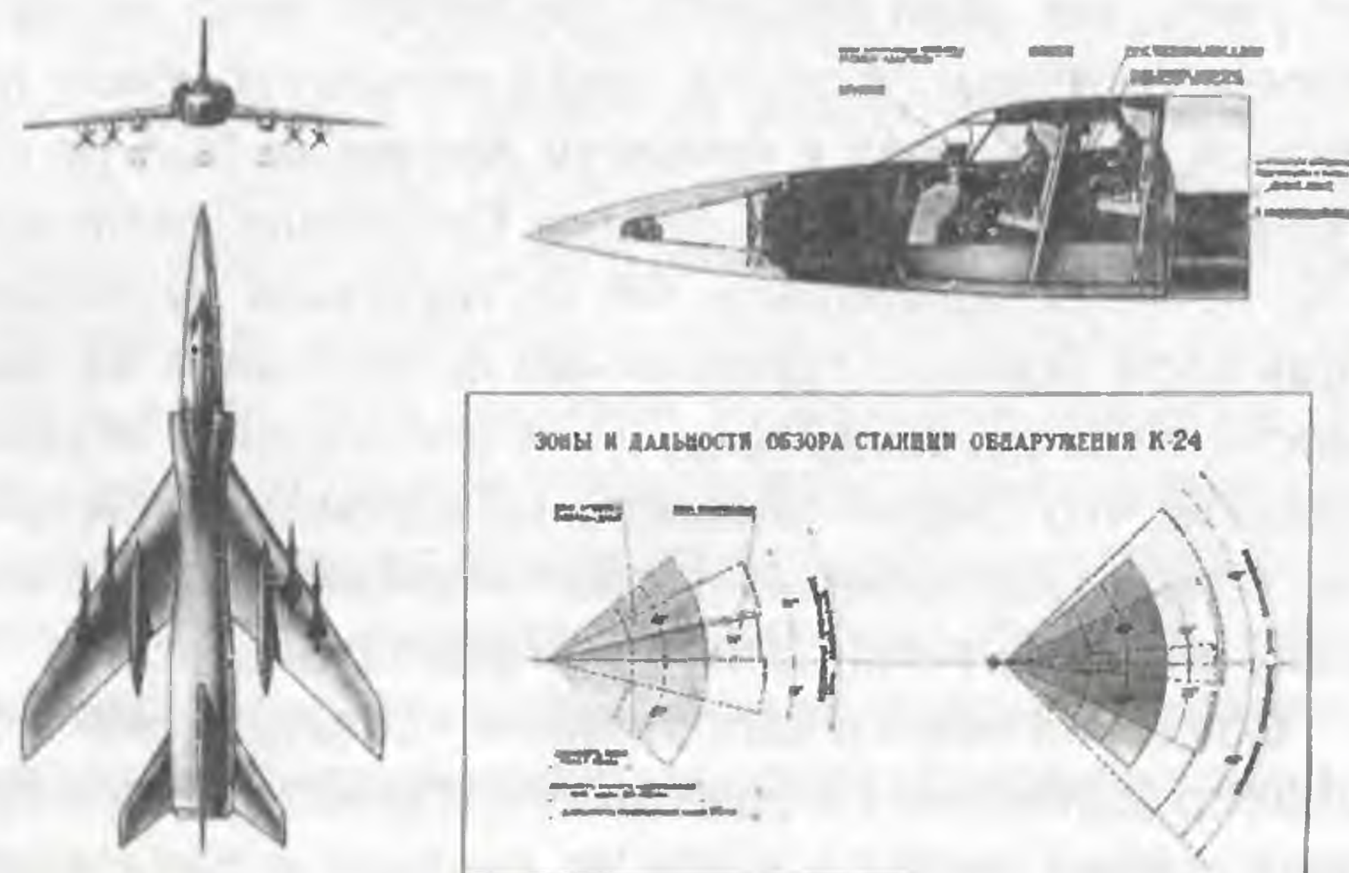
ПОДВЕСКА РАКЕТ ПВО ПОД САМОЛЕТ ТУ-28
