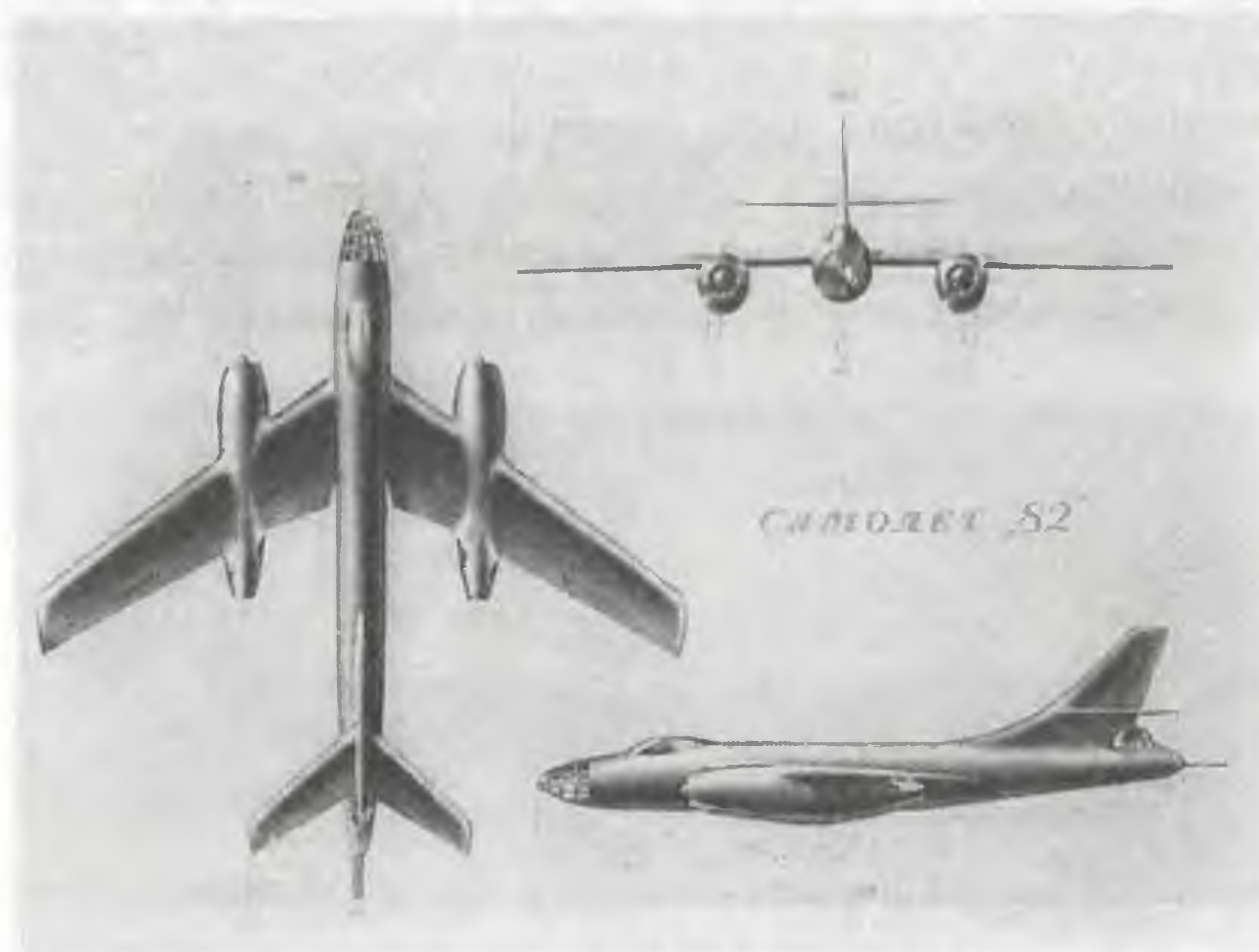
Общий вид самолета Ту-82
