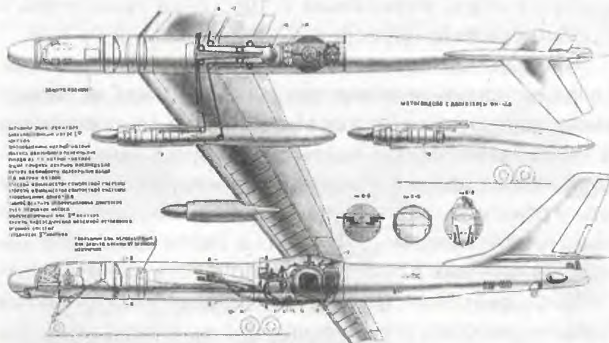
ЭКСПЕРИМЕНТАЛЬНЫЙ САМОЛЕТ ТУ-119 С ЯСУ НК-14А
