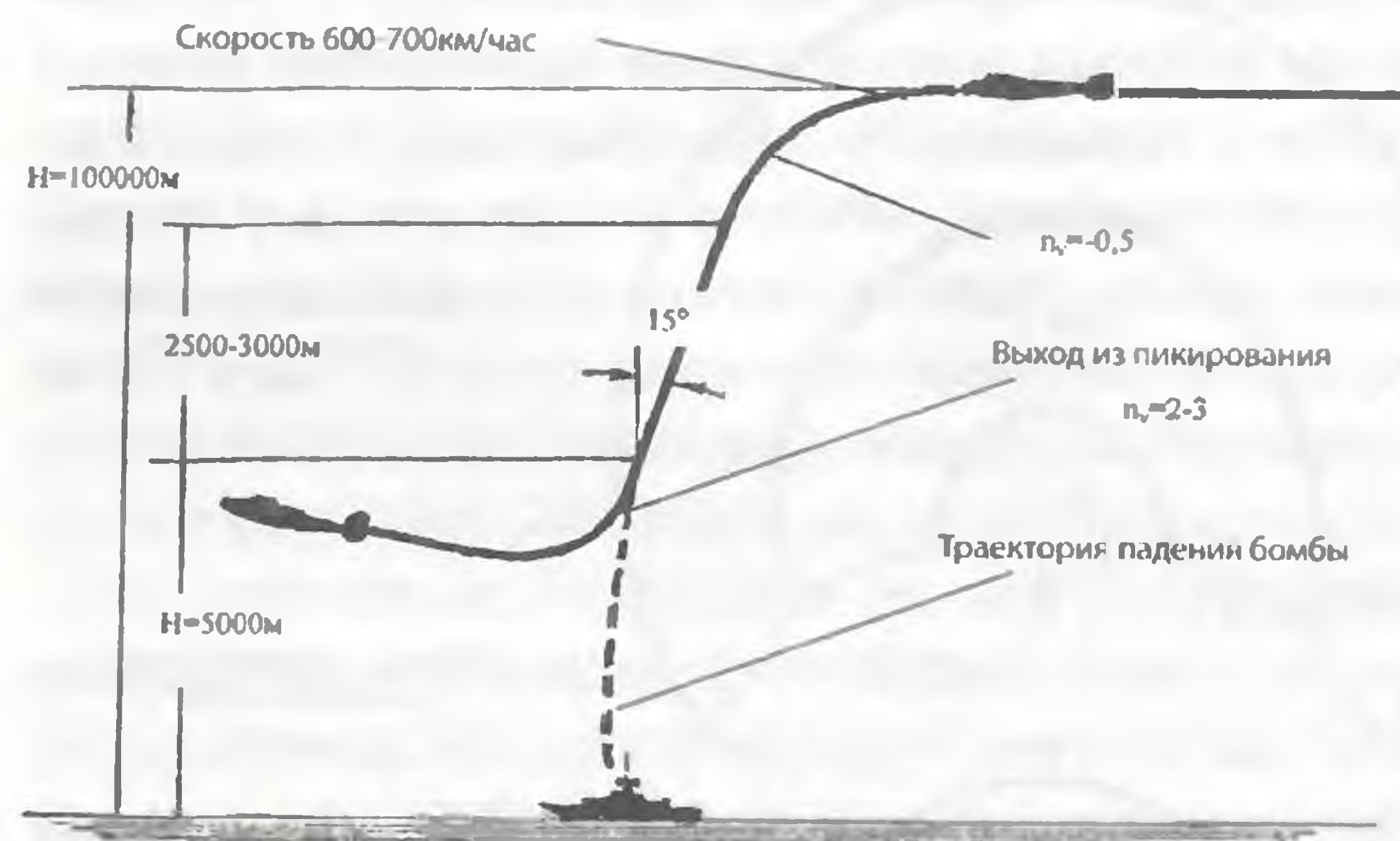
Схема бомбометания с пикирования
