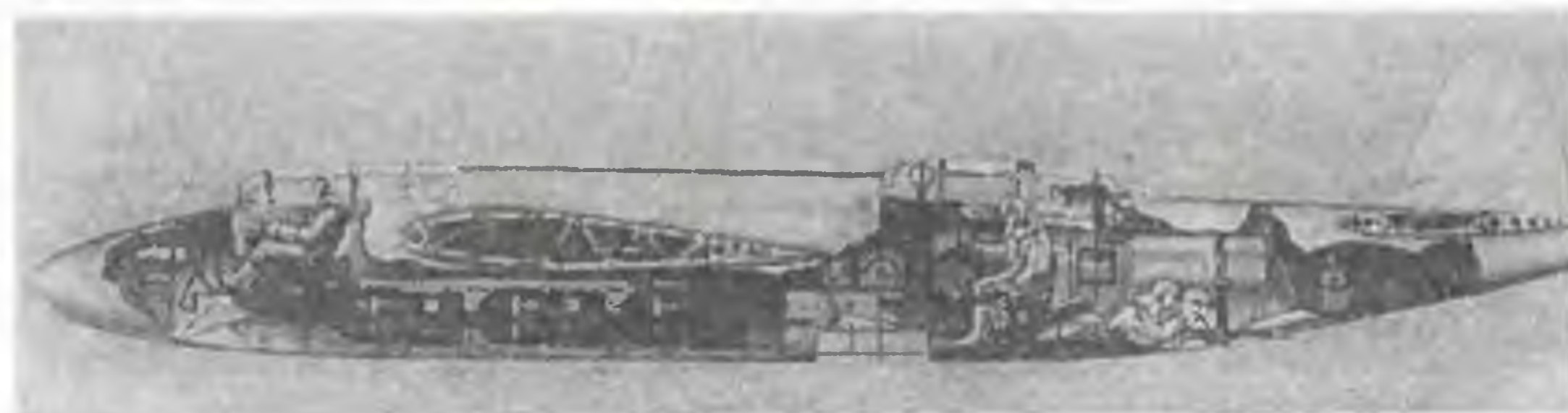
Компоновка самолета «103»
