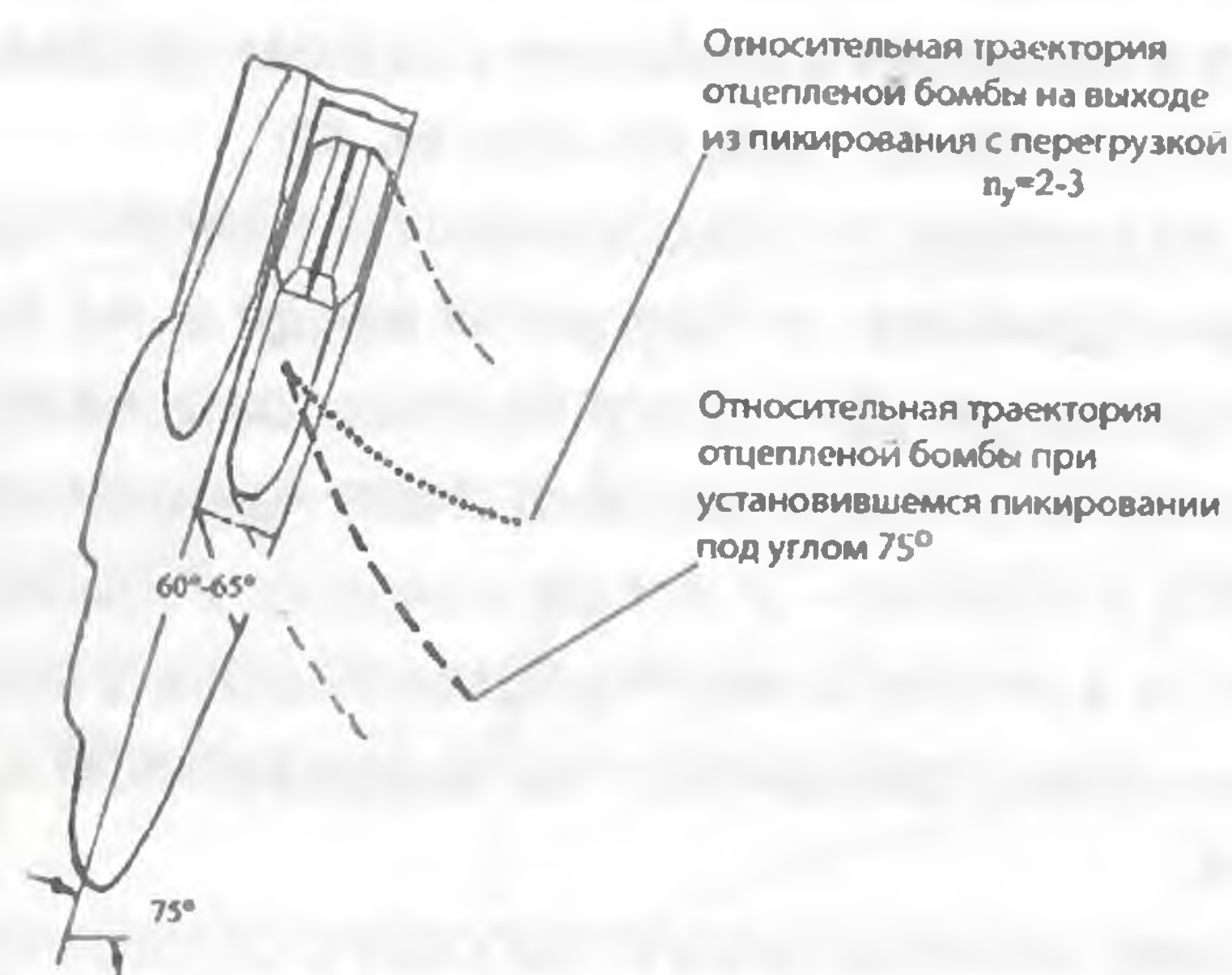
Движение центра масс бомбы относительно самолёта на пикировании
