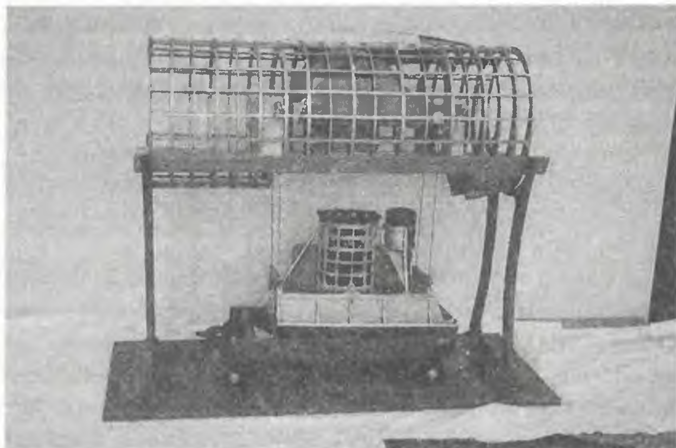
Макетирование установки реактора на самолет
