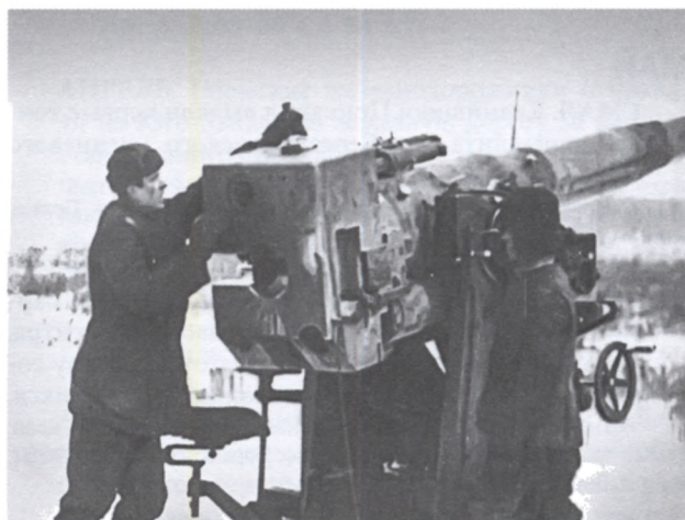
Испытание 122-мм дивизионной гаубицы М-30 образца 1938 г.
