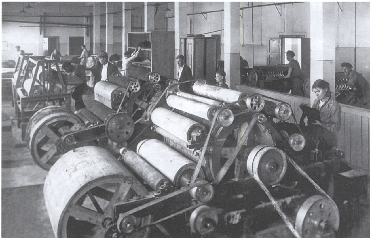
Наладили не только выпуск моторов, но и валенок. Пимокатные станки в цехе 71 завода № 19
