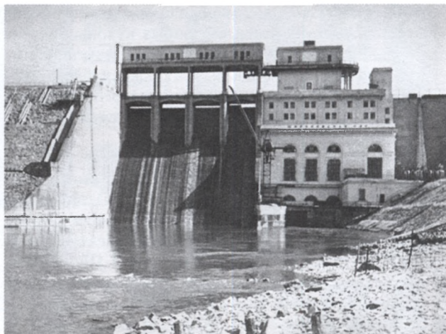
Широковская ГЭС. Фото 1950-х гг.
