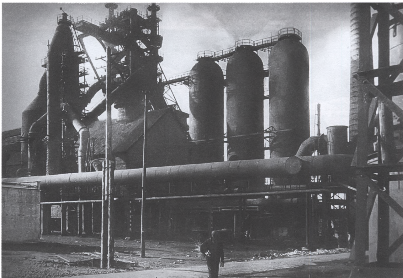
Домна № 2, построенная за семь месяцев – в рекордно короткий срок
