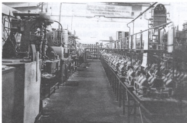
Поточная линия по сборке карбюраторов на заводе № 33
