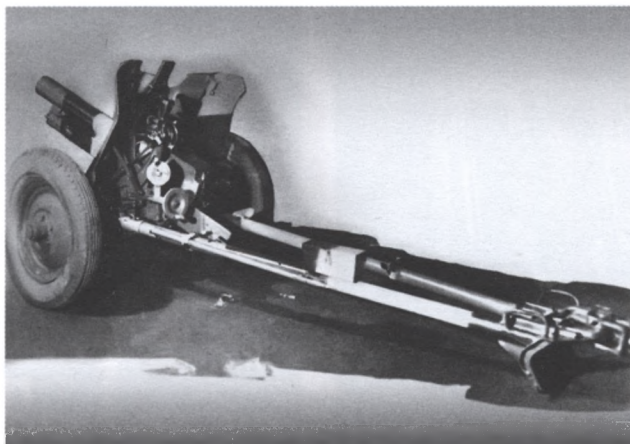
76-мм полковая пушка образца 1943 г. (ОБ-25). Изготовлена по проекту ОКБ-172 НКВ. Калибр 76 мм, вес снаряда 6,23 кг, дальность макс. 4400 м, вес 600 кг
