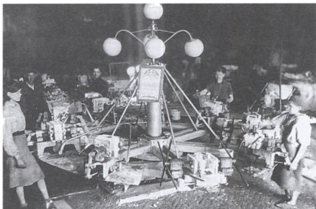
Конвейер карусельного типа в литейном цехе завода № 33
